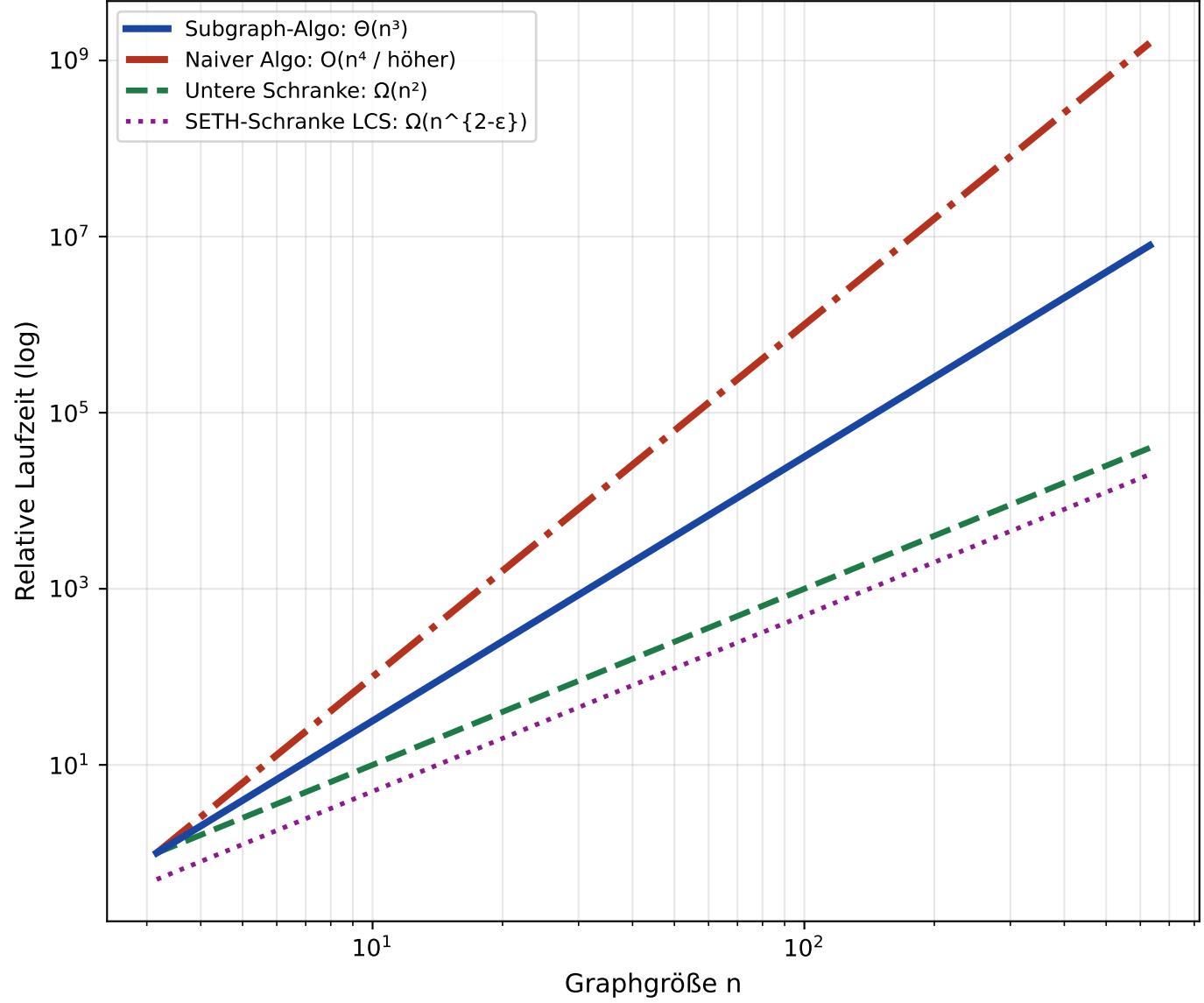
Komplexitätsvergleich: Subgraph- Algo vs. Naive Verfahren
