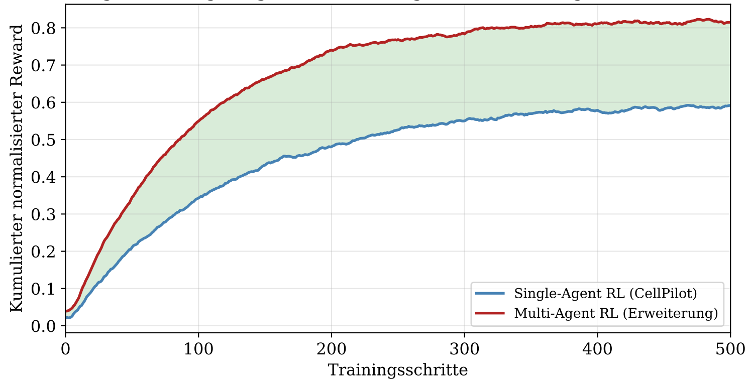
Vergleich: Single-Agent vs. Multi-Agent RL (Konvergenzsimulation)
