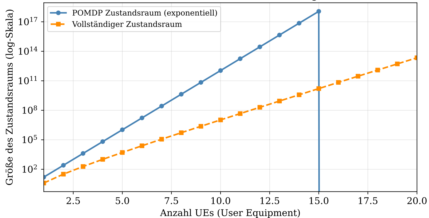
Wachstum des POMDP-Zustandsraums mit steigender UE-Anzahl
