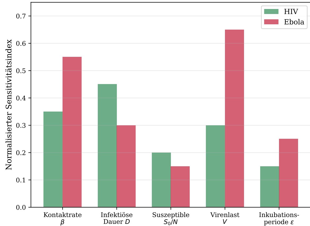
Parameter-Sensitivität für R_0
