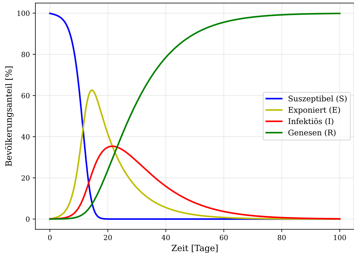
Ebola SEIR-Modell
