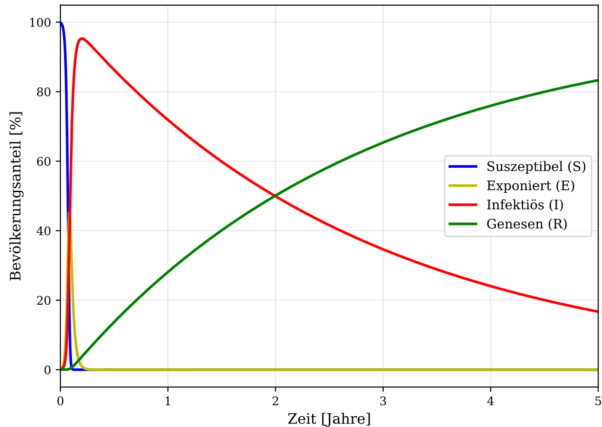
HIV SEIR-Modell (Unbehandelt)
