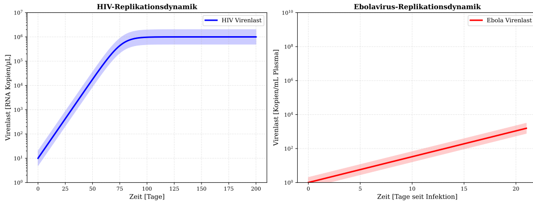
Figure 1: Within-Host-Virenreplikationsdynamik für HIV und Ebola. Das linke Panel zeigt die logistischen Wachstumskurve von HIV mit charakteristischen Parametern: Wachstumsrate r_{\text{HIV}} \approx 0,15 \text{ Tag}^{-1} , resultierende Virenplateaus bei \approx 10^6 RNA-Kopien/ \mu\text{L} nach \approx 200 Tagen. Das rechte Panel illustriert Ebolavirenreplikation mit schnellerem Wachstum ( r_{\text{Ebola}} \approx 0,35 \text{ Tag}^{-1} ), höherer Plateauvirenlast ( 10^9 Kopien/mL) und kürzerer Virenausscheide-Periode (ca. 21 Tage). Die blaue/rote Füllung zeigt die Variabilität um 2-fach um den Median. Biologische Interpretation: HIV etabliert ein chronisches Quasi-Gleichgewicht mit moderater Virämie und jahrelanger Persistenz. Ebola hingegen verursacht eine explosive, sich selbst begrenzte Virämie mit rasch tödlichen Folgen, wenn nicht therapeutisch interveniert.
