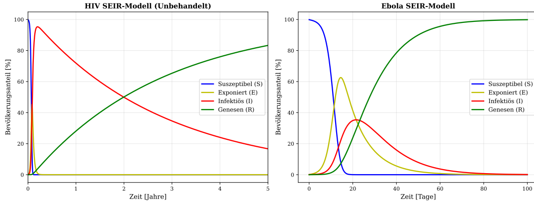
Figure 3: Bevölkerungs-Ebene Kompartimentdynamik für HIV und Ebola. Linkes Panel: HIV-SEIR mit langsamem Infektionsübergang ( \sigma = 0,1 \text{ Tag}^{-1} , d.h. 10 Tage Inkubation) und sehr langsamer Genesungsrate ( \gamma = 0,001 \text{ Tag}^{-1} , d.h. 1000 Tage Infektiosität ohne Therapie). Die Epidemie breitet sich über Jahre aus und erreicht kein Plateau. Rechtes Panel: Ebola-SEIR mit kurzer Inkubation (10 Tage) und kurzer Infektiosität (10 Tage). Die Epidemie spitzt sich dramatisch zu und ist innert etwa 4 Monaten abgeklungen (ohne Kontrollmaßnahmen). Die unterschiedliche Zeitskala (1 Jahr für HIV vs. 100 Tage für Ebola) verdeutlicht die epidemiologischen Unterschiede. Präventiv-strategische Folgerung: HIV erfordert langfristige, dauerhafte Interventionen; Ebola erfordert intensive kurzfristige Kontrollmaßnahmen.
