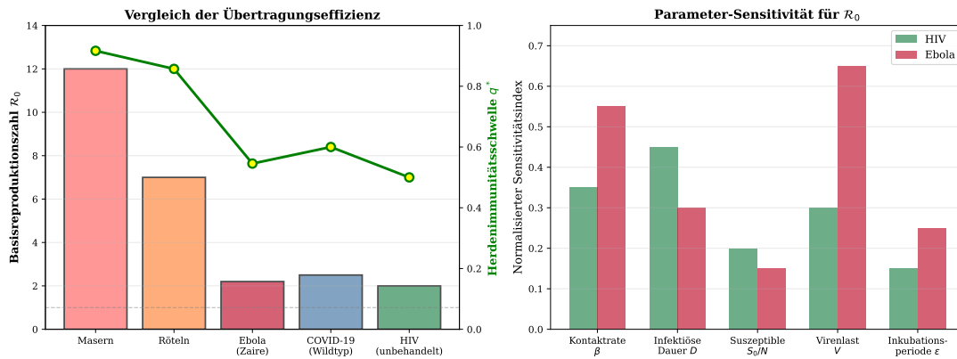
Figure 2: Vergleichende Analyse der Basisreproduktionszahl und ihrer Parameter. Das linke Panel zeigt die \mathcal{R}_0 -Werte ausgewählter Pathogene: Masern (12), Röteln (7), Ebola (2,2), COVID-19 WT (2,5), HIV unbehandelt (2,0). Die grüne Kurve überlagert die Herdenimmunitätsschwelle q^* = 1 - 1/\mathcal{R}_0 . Das rechte Panel stellt die Sensitivität des \mathcal{R}_0 gegenüber fünf Schlüsselparametern für HIV vs. Ebola dar. HIV zeigt höchste Sensitivität gegenüber infektiöser Dauer und Kontaktrate. Ebola ist stark von Virenlast und Kontaktrate abhängig. Klinische Implikation: Interventionen sollten auf den Parametern mit höchster Sensitivität ansetzen – für HIV: Therapie (Virenlast), für Ebola: Kontaktreduktion und Isolation.
