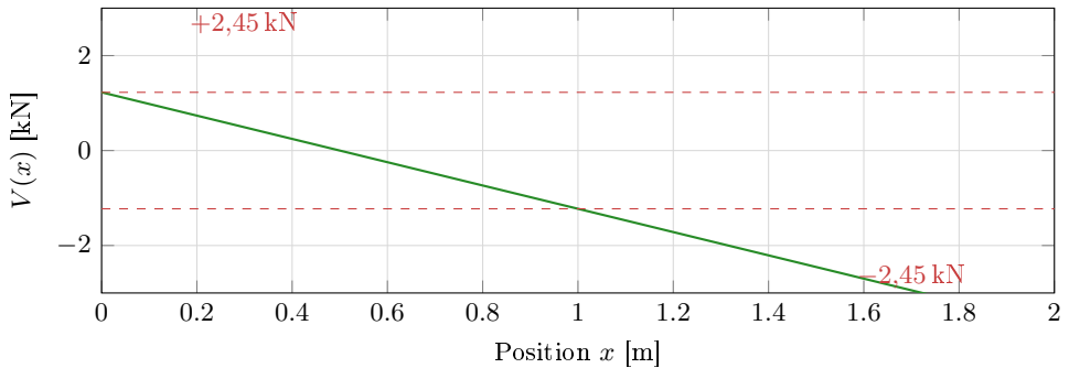
Querkraftlinie
