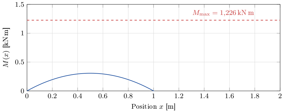
Momentenlinie
