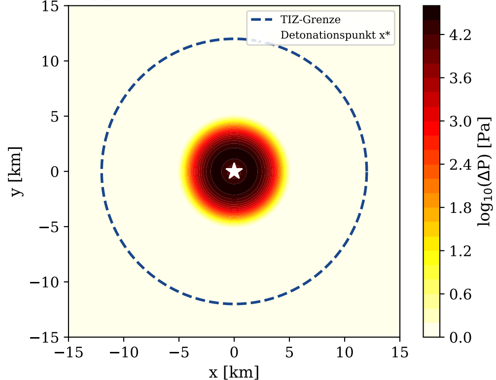
(b) 2D-Druckwellenfeld bei t = 2.0 s
