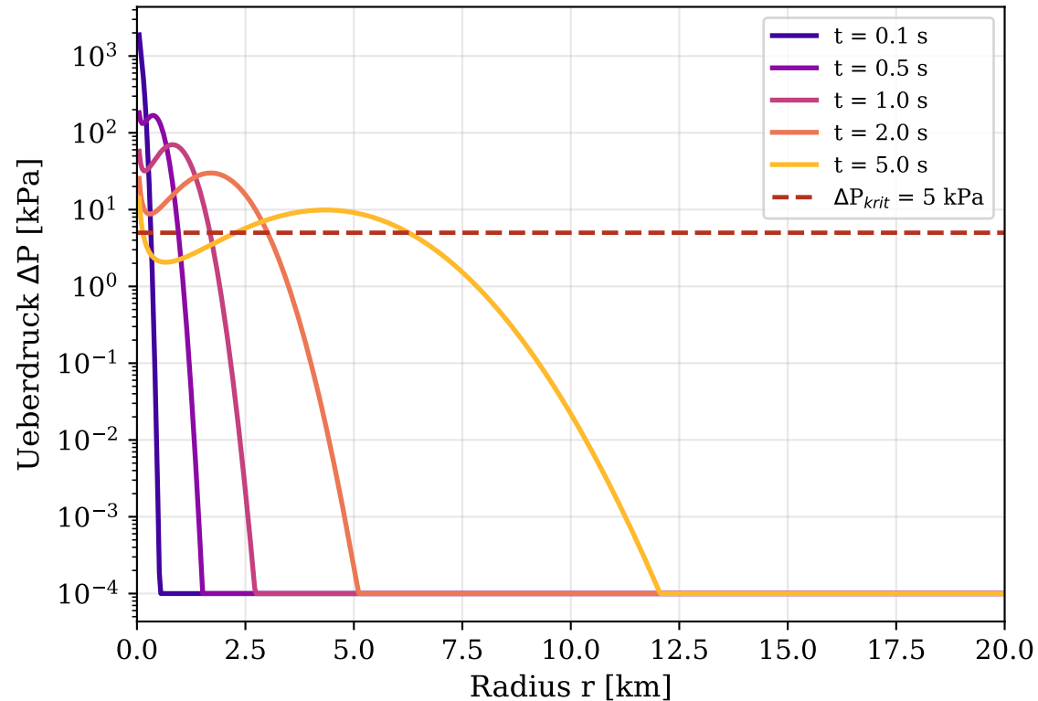
(a) Radiales Druckprofil zu verschiedenen Zeiten
