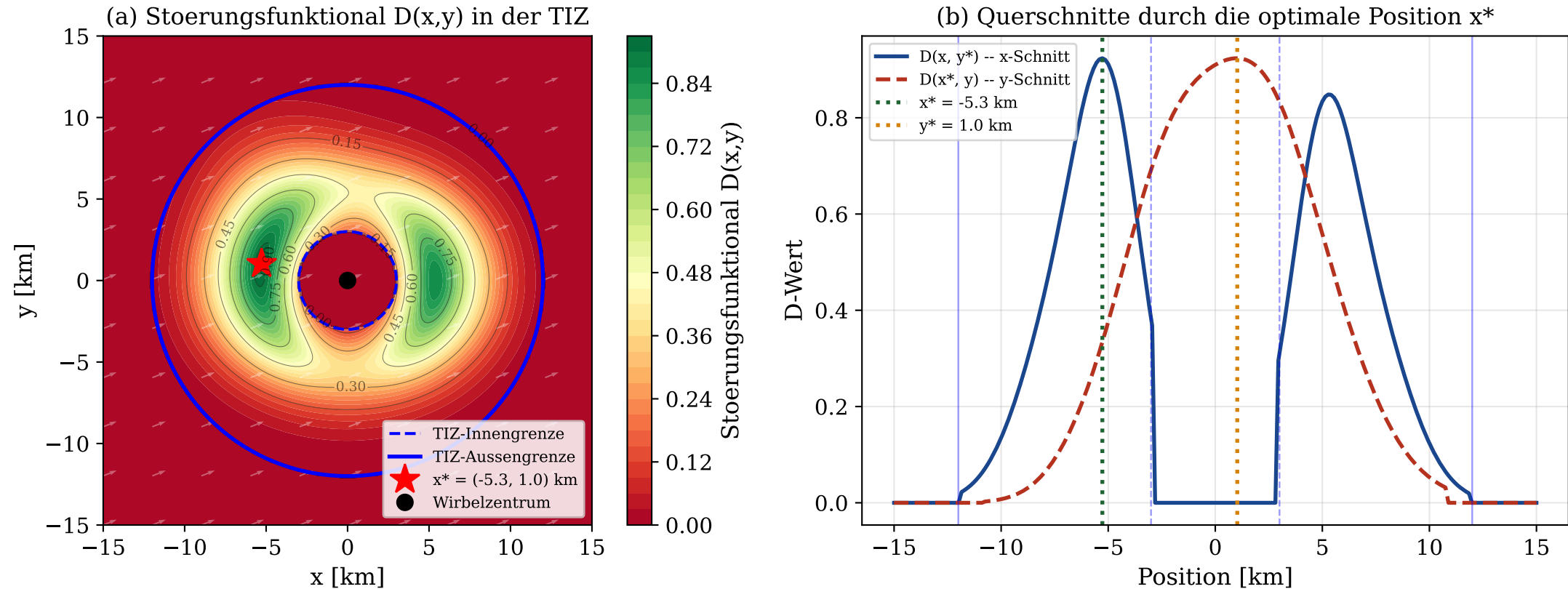
Abbildung 5: Optimale Detonationsposition x^* im Störungsfunctional D(x,y) und Querschnitte durch das globale Maximum in der TIZ
