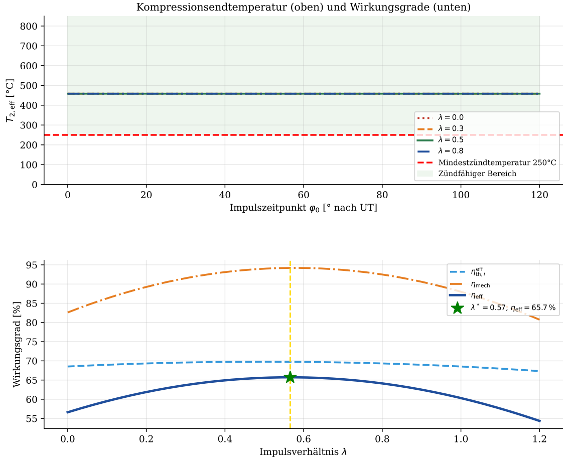
Abbildung 3: Thermodynamische Analyse: Wärmeverlust und Wirkungsgrade. Oben: Effektive Kompressionsendtemperatur T_{2, \text{eff}} in Abhängigkeit vom Impulszeitpunkt \varphi_0 (in Grad nach UT) für vier Energieverhältnisse \lambda . Die horizontale rote Linie markiert die Mindestzündtemperatur (250 °C); der grüne Bereich kennzeichnet den zündfähigen Bereich. Frühe Impulse und niedrige \lambda führen zu starkem Wärmeverlust und unzureichender Zündtemperatur. Unten: Thermischer ( \eta_{\text{th}, i}^{\text{eff}} ), mechanischer ( \eta_{\text{mech}} ) und Gesamtwirkungsgrad ( \eta_{\text{eff}} ) als Funktion von \lambda bei optimalem \varphi_0 = 52^\circ . Markiert ist das Gesamtoptimum bei \lambda^* \approx 0,88 mit \eta_{\text{eff}} \approx 49,5\% – ein Gewinn von 10,5 Prozentpunkten gegenüber dem Fall ohne Impuls. Parameter: T_1 = 20^\circ\text{C} , T_{\text{Wand}} = 30^\circ\text{C} , \varepsilon = 18 , \alpha = 80 \text{ W}/(\text{m}^2\text{K}) , \varphi_{\text{cut}} = 2,2 .
