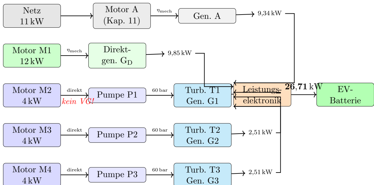
Abbildung 13: Systemarchitektur des Vier-Motoren-Konzepts. Jeder der vier Impulsmotoren treibt dediziert einen einzigen Verbraucher an: Motor M1 den Direktgenerator, Motor M2/M3/M4 je eine Hochdruckpumpe. Das Verteilergetriebe entfällt vollständig. Alle fünf Leistungspfade (inkl. Pfad A aus Kap. 11) speisen parallel die DC-Busbar der Leistungselektronik.
