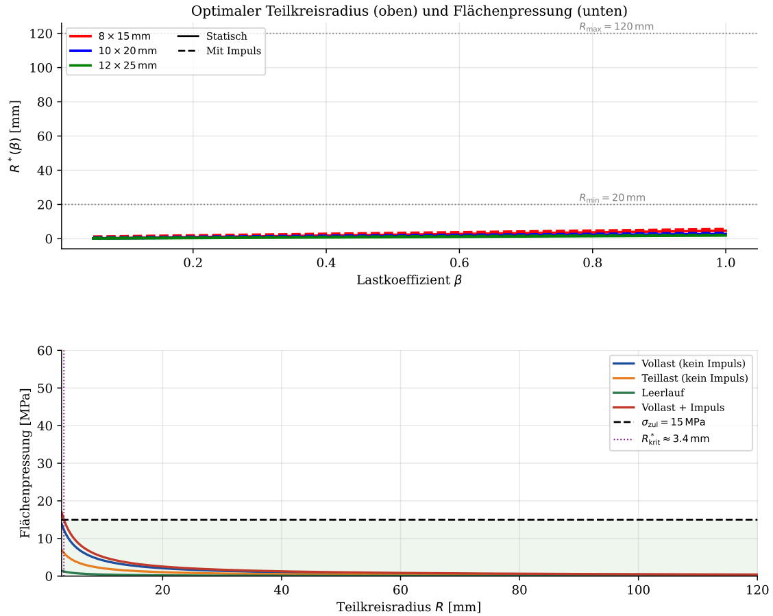
Abbildung 7: Optimaler Teilkreisradius und Flächenpressung unter statischer und dynamischer Belastung. Oben: Mindest-Teilkreisradius R^*(\beta) als Funktion des Lastkoeffizienten \beta für drei Bolzengrößen (rot: 8 \times 15 mm, blau: 10 \times 20 mm, grün: 12 \times 25 mm). Durchgezogene Linien: statischer Lastfall; gestrichelte Linien: dynamischer Lastfall mit Impuls ( \lambda^* = 0,52 ). Die horizontalen Linien bei R = 20 mm und R = 120 mm markieren praxisübliche Bauraumbeschränkungen. Alle R^* -Werte liegen weit unterhalb, d. h. die Festigkeit ist nicht limitierend. Unten: Flächenpressung p(R) für alle drei Lastfälle (Vollast rot, Teillast orange, Leerlauf grün) mit und ohne Impuls. Die schwarze horizontale Linie bei \sigma_{zul} = 15 MPa trennt den zulässigen (grün hinterlegt) vom Überlastbereich (rot hinterlegt). Die vertikale Linie bei R_{krit}^* \approx 3,4 mm markiert den kritischsten Fall (Vollast + Impuls). Praxisübliche Radien ( R \geq 20 mm) liegen weit im sicheren Bereich. Parameter: N = 3 Bolzen, \sigma_{zul} = 15 MPa, M_{mot,max} = 25 N m, M_{imp} = 5,5 N m.
