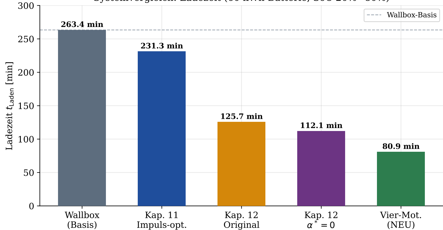
Systemvergleich: Ladezeit (60 kWh-Batterie, SoC 20%→80%)
