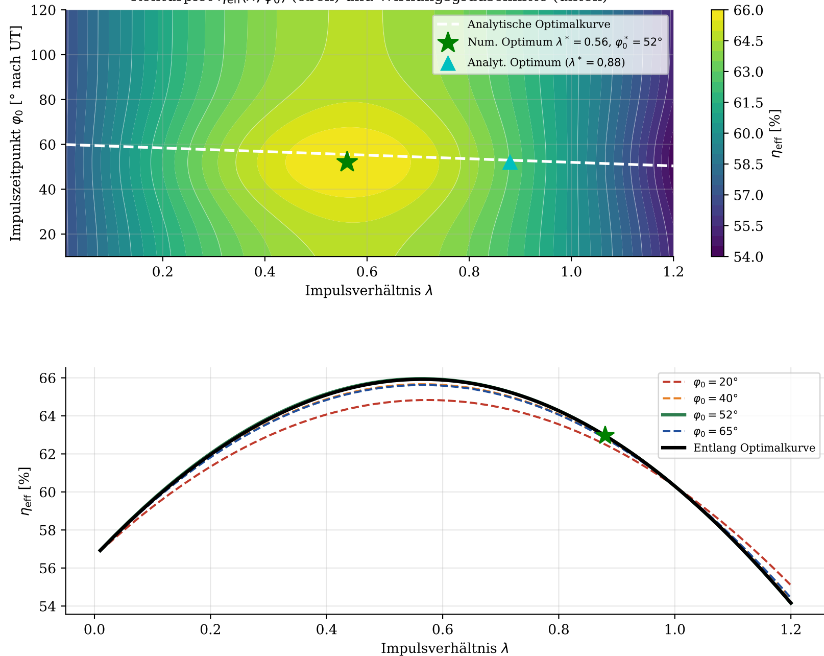
Konturplot \eta_{\text{eff}}(\lambda, \varphi_0) (oben) und Wirkungsgradschnitte (unten)
