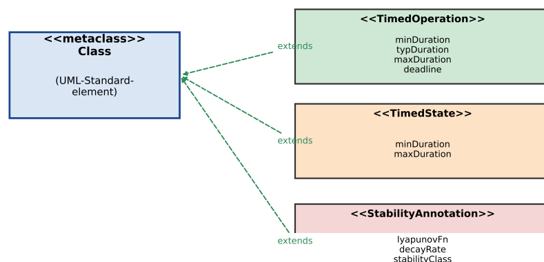
Abbildung 3.1.1: Struktur eines UML-Profiles mit Zeit-Annotationen
