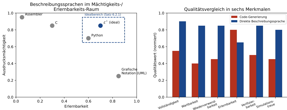
Abbildung 6.2.1: Links: Beschreibungssprachen im zweidimensionalen Raum von Ausdrucks-mächtigkeit und Erlernbarkeit. Der blau gestrichelte Idealbereich kennzeichnet das Optimum nach Satz 6.2.1: hohe Mächtigkeit bei gleichzeitig guter Erlernbarkeit. Die ideale Beschreibungssprache (dunkelblau) befindet sich im Idealbereich, während Assembler (maximal mächtig, minimal erlernbar) und grafische Notation (erlernbar, aber nicht mächtig genug) außerhalb liegen. Rechts: Qualitätsvergleich zwischen Code-Generierung aus graphischer Modellierung und direkter Beschreibungssprache in sechs Merkmalen. Die direkte Beschreibungssprache dominiert in allen Dimensionen.
