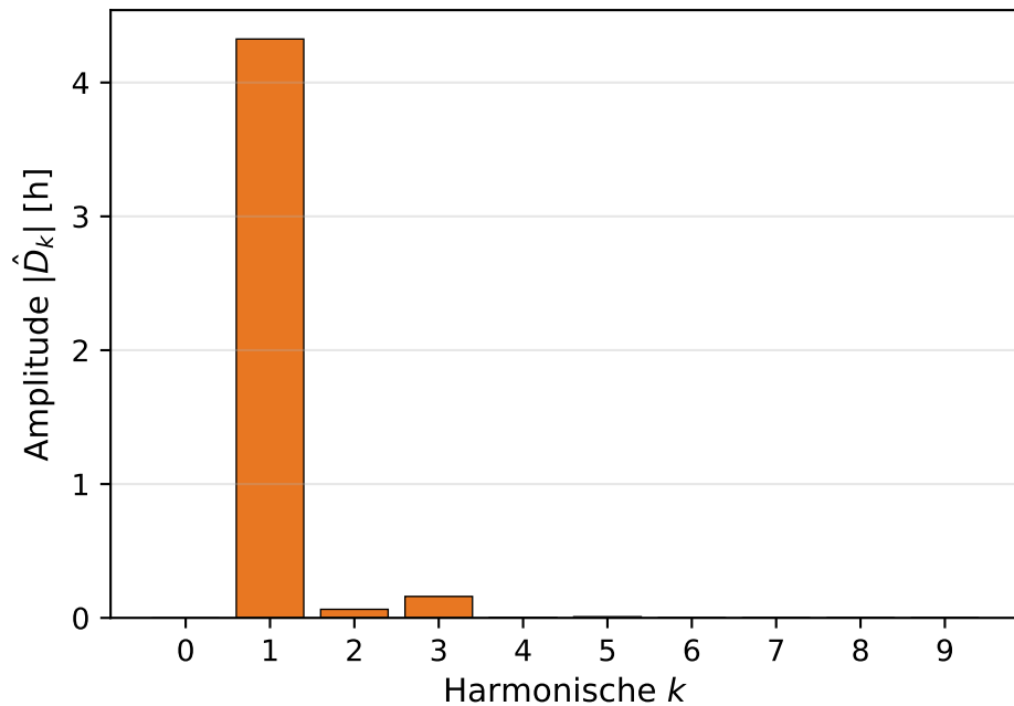
(c) Fourier-Spektrum der Tageslänge
