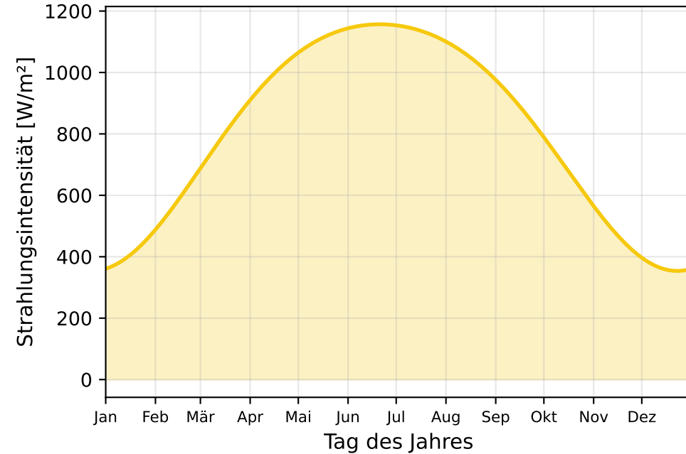
(d) Solare Mittagsstrahlung (Bielefeld)
