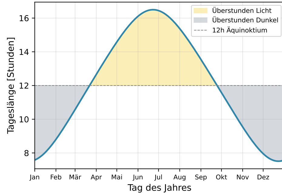
(b) Tageslänge D(t) (Bielefeld, \varphi = 52^\circ\text{N} )
