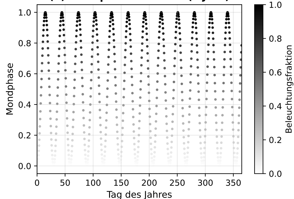
(b) Mondphasen-Verlauf (1 Jahr)
