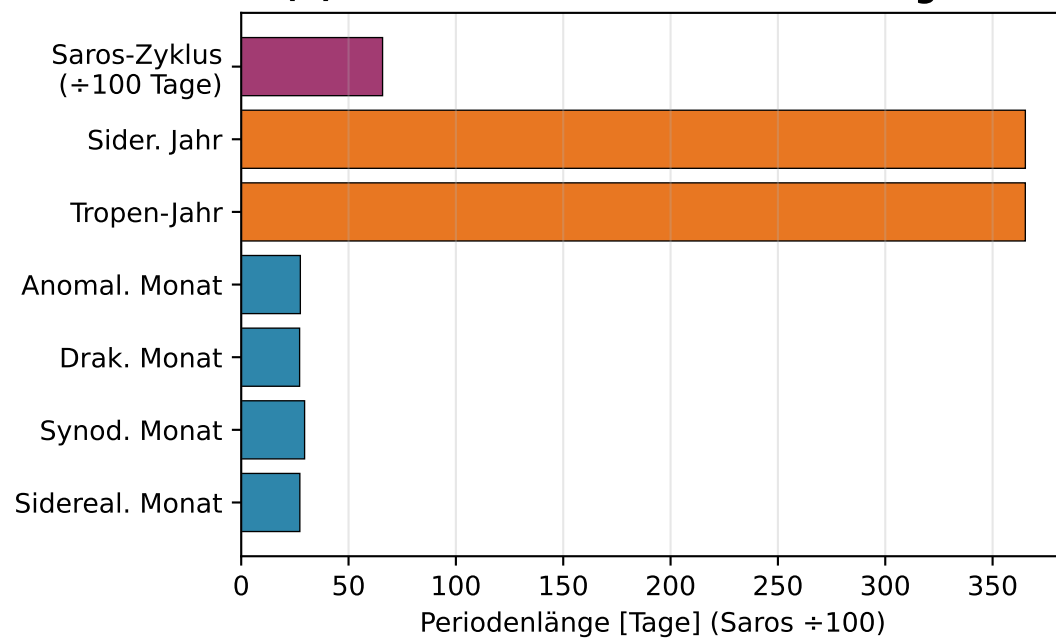
(d) Astronomische Perioden im Vergleich
