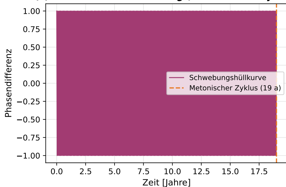
(c) Mond-Sonne-Schwebung (Metonischer Zyklus)
