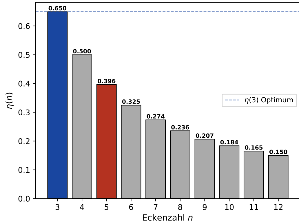
Effizienzmaß \eta(n) nach Polygon-Typ
