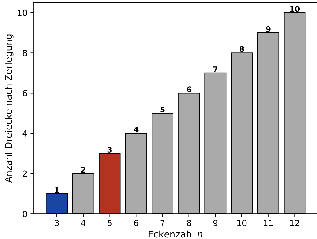
Dreiecksanzahl n - 2 bei Fächerzerlegung
