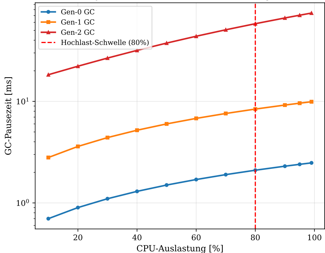
Python GC-Pausen vs. CPU-Auslastung
