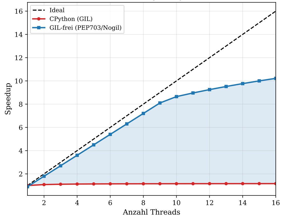
GIL-Effekt: Skalierung bei Python-Threads
