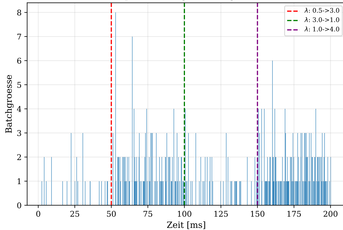
Batchgrössenverteilung nach Laststufe
