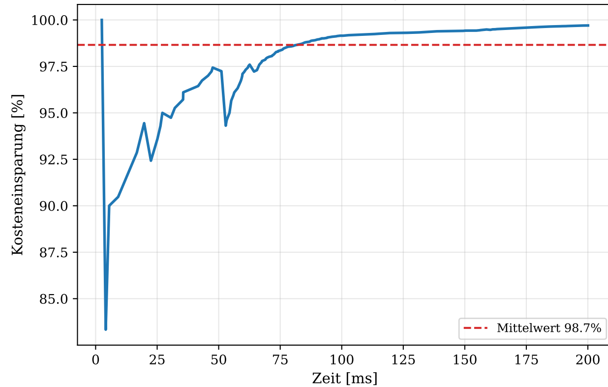
Kumulative Kosteneinsparung durch Batching
