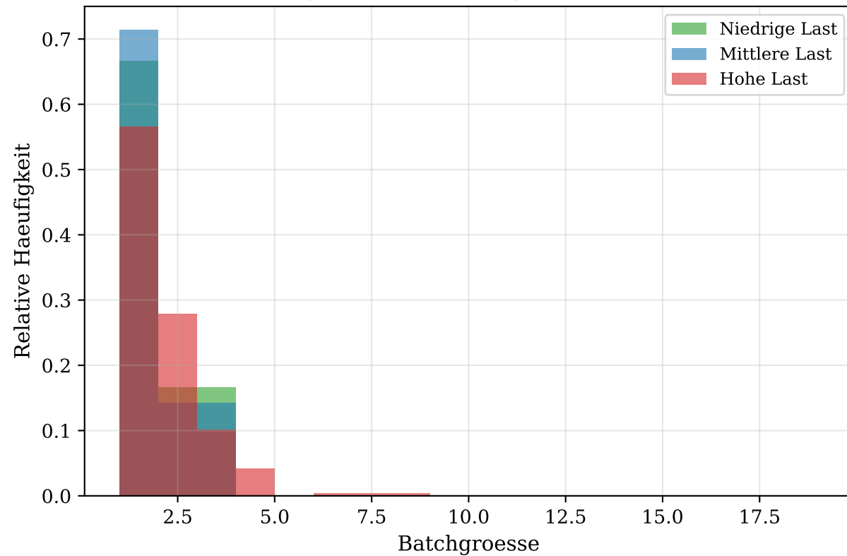
Batchgrössenverteilung nach Laststufe
