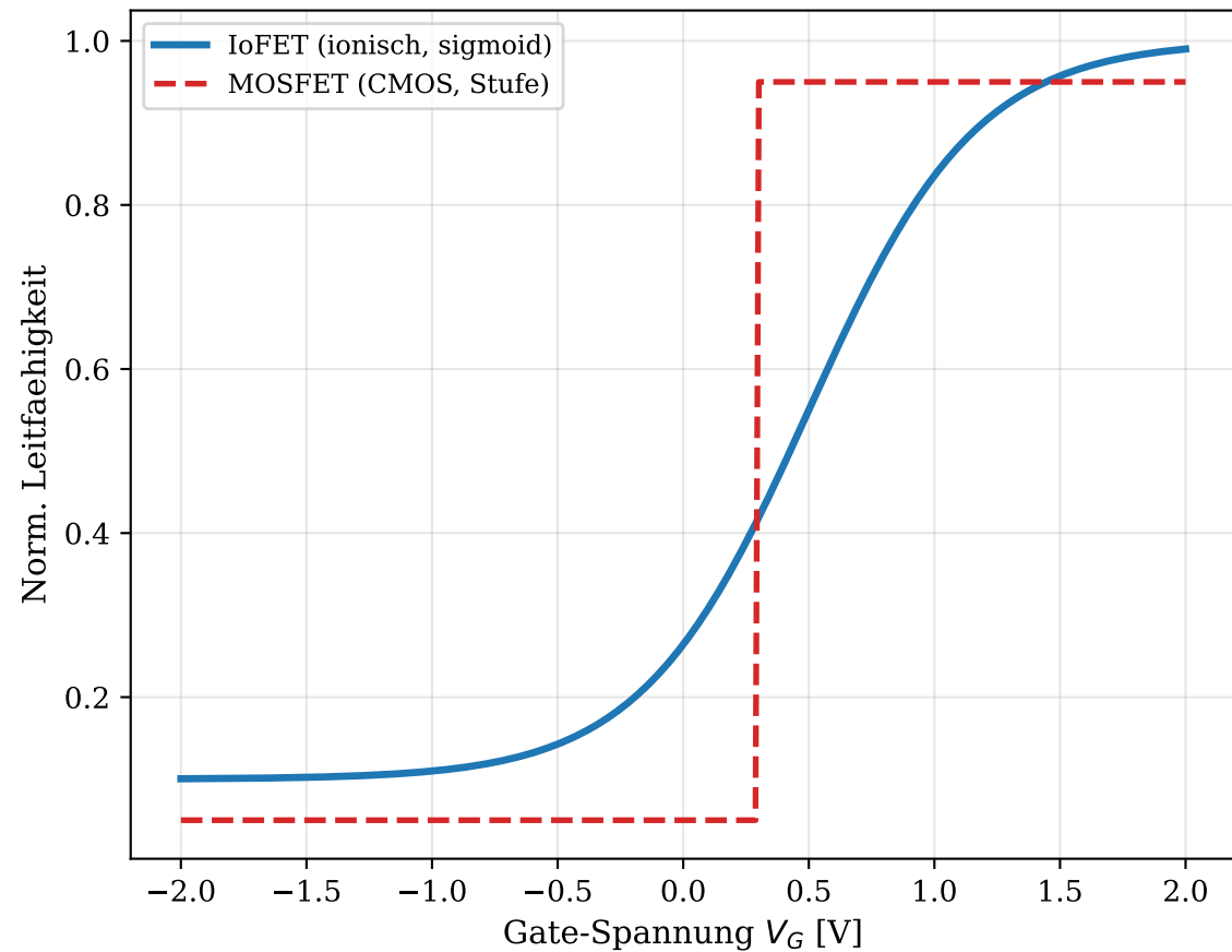
IoFET vs. MOSFET: Transfercharakteristik
