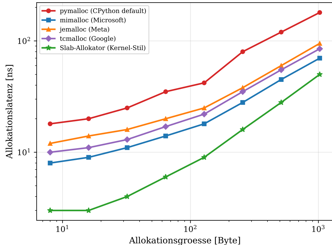
Allokator-Vergleich: Latenz vs. Objektgrösse
