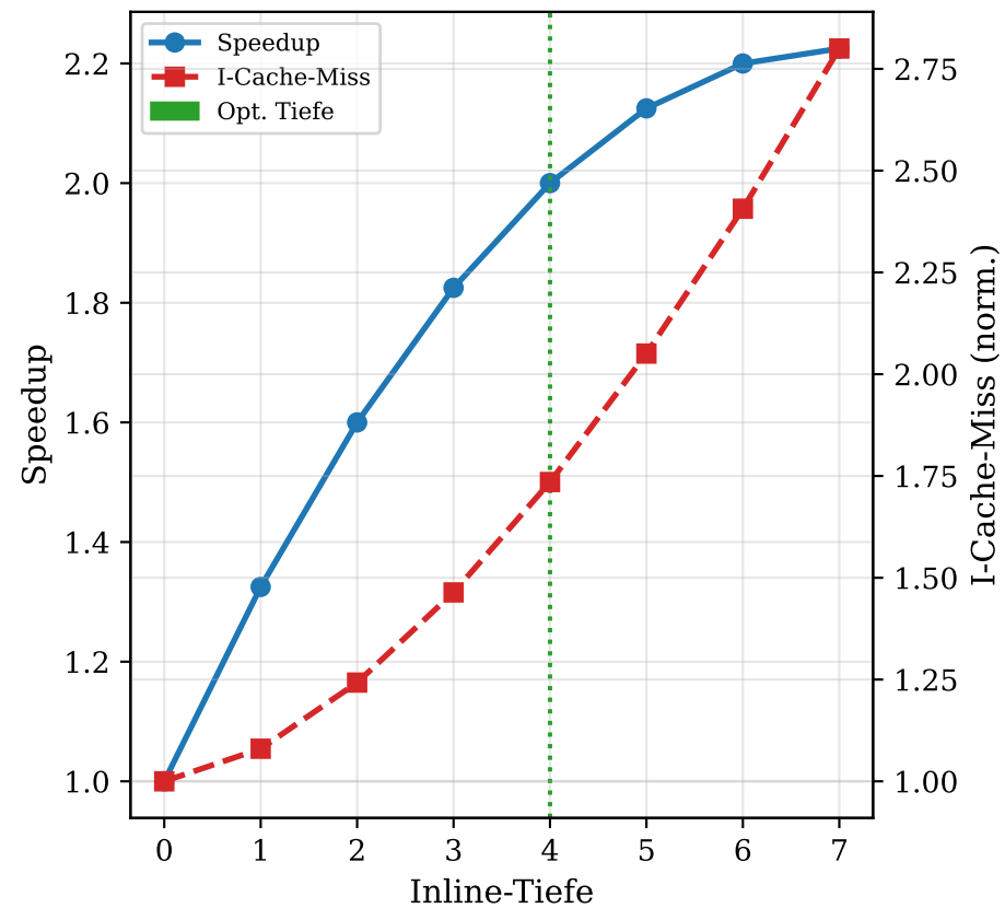
Inlining-Tiefe: Speedup vs. I-Cache-Druck
