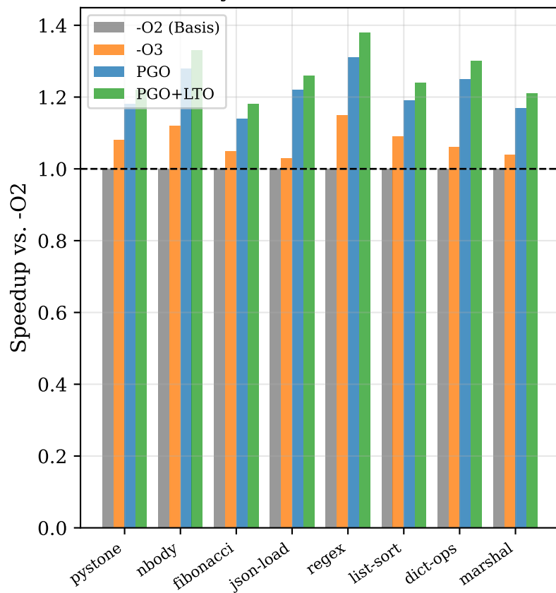
PGO / LTO Effekte auf Python-Benchmarks
