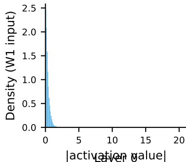
Layer 0
