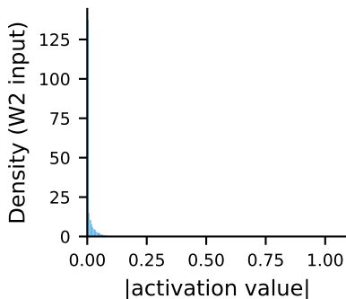
Layer 0
