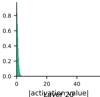
Layer 20
