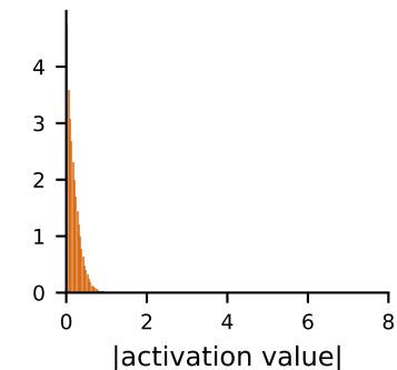
Layer 39
