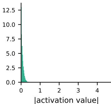
Layer 20
