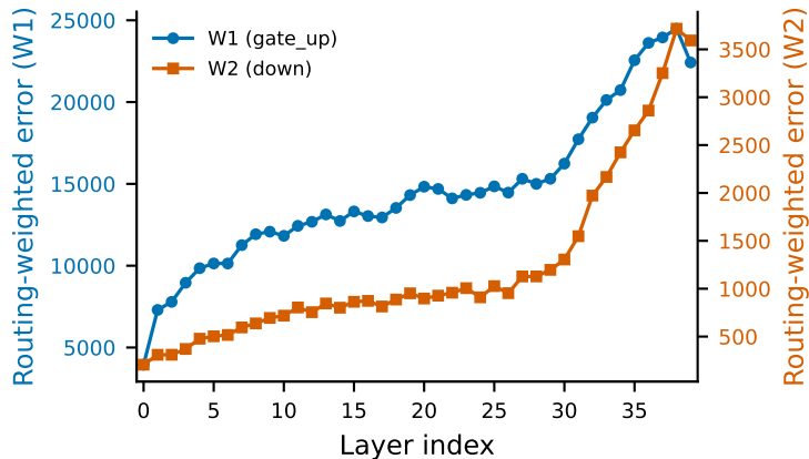
(d) Routing-weighted NVFP4 error by depth ( \sum rw \times MAE )
