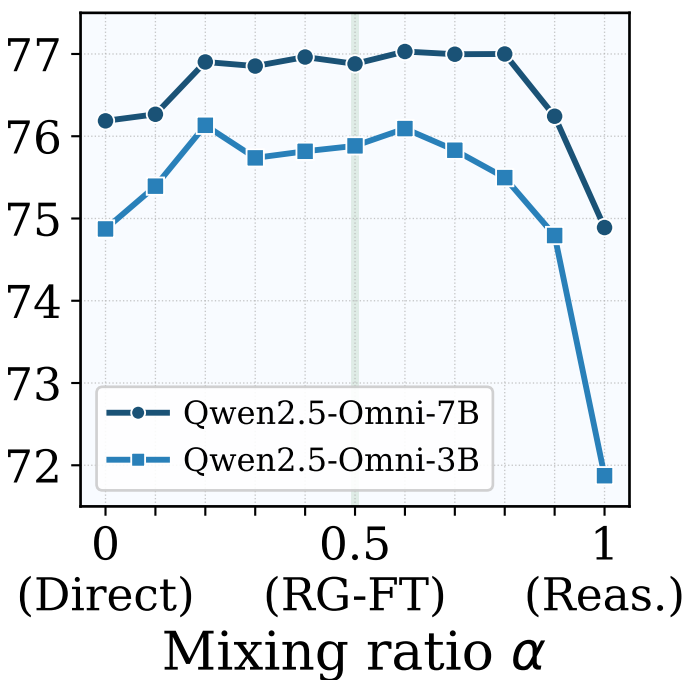
SLU-F1
