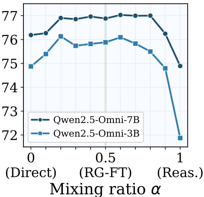
SLU-F1
