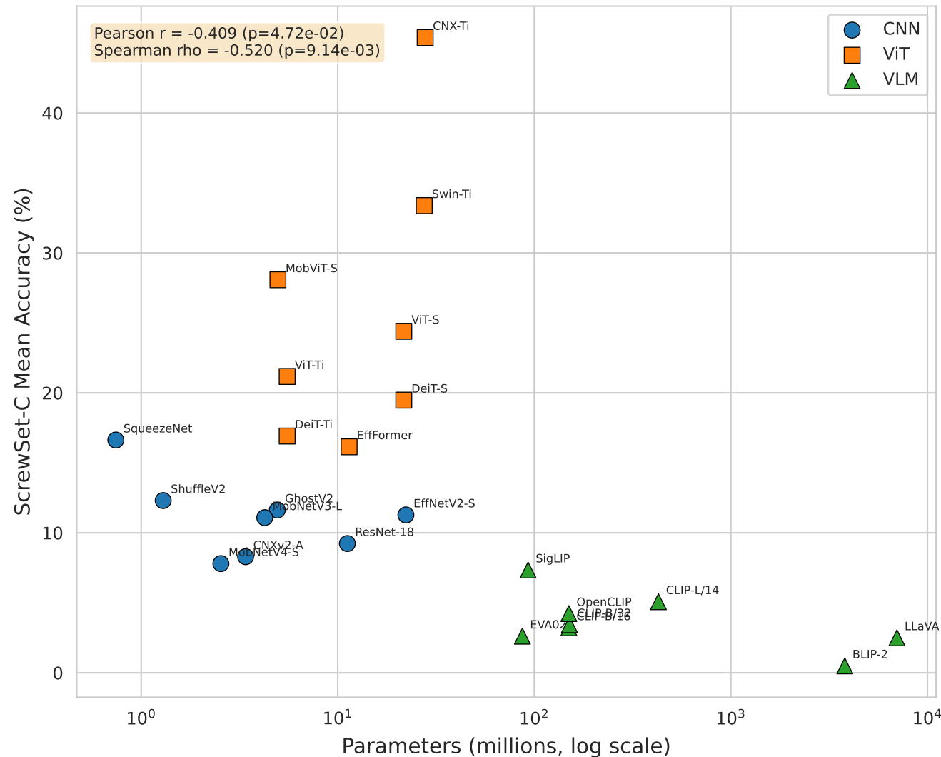
A1. Parameter Count vs Corruption Robustness
