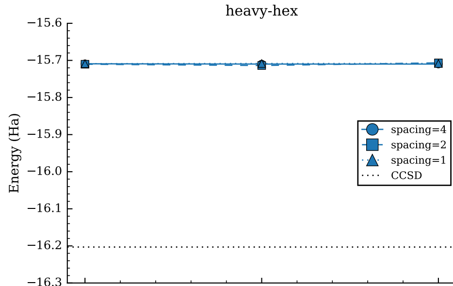
H30 chain — pairs_ab parameter sweep
