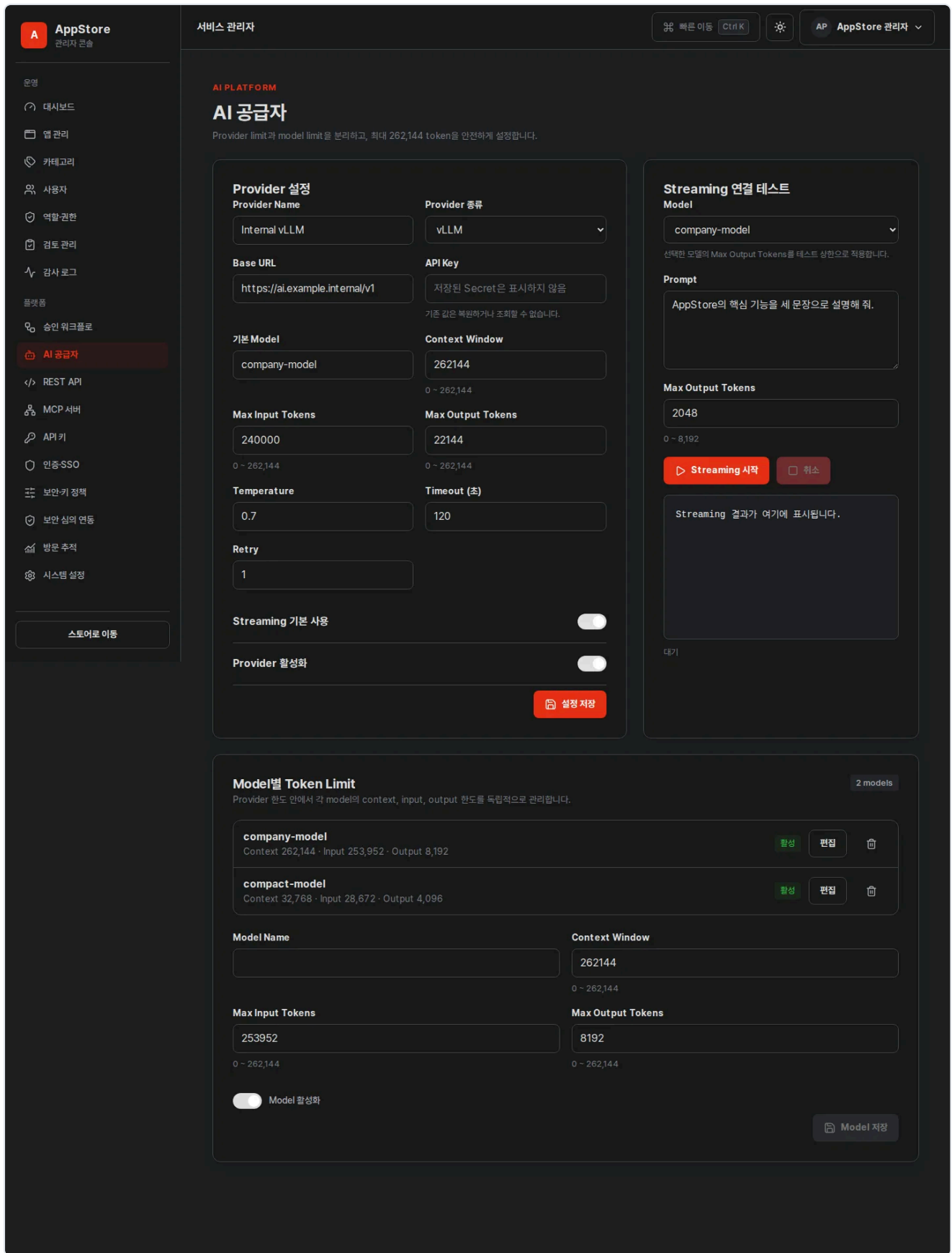
AI 공급자 — provider와 모델별 token 한도, streaming 설정
