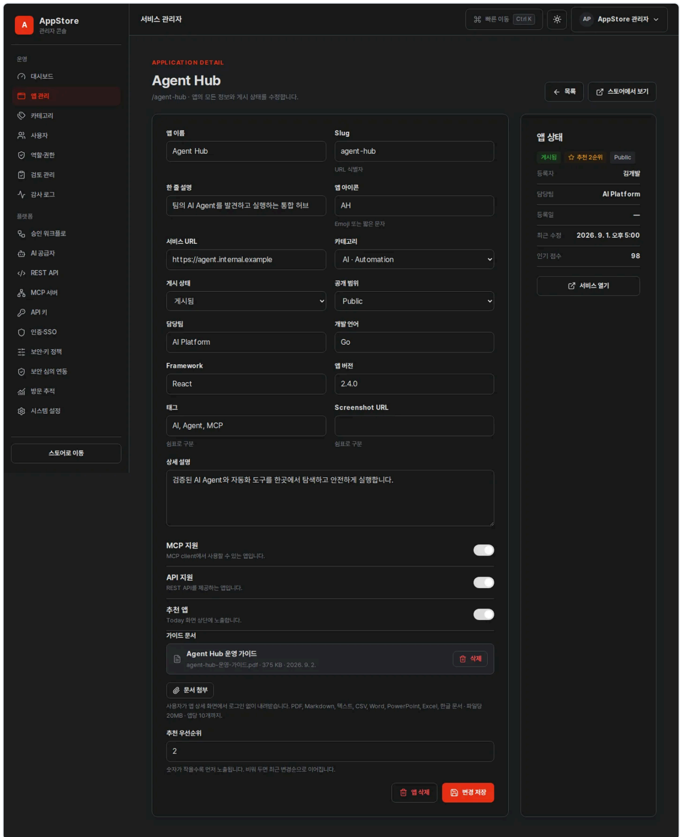
앱 상세 — 앱의 모든 정보와 게시 상태를 수정하는 관리자 화면
