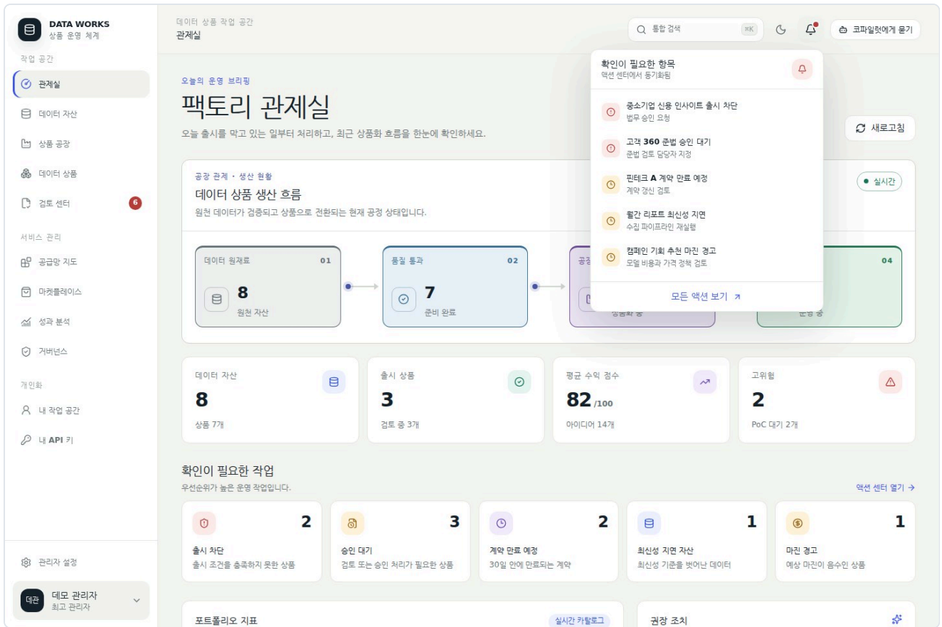
알림 센터 — 승인 대기와 출시 차단 등 운영 신호를 모아 보여준다
