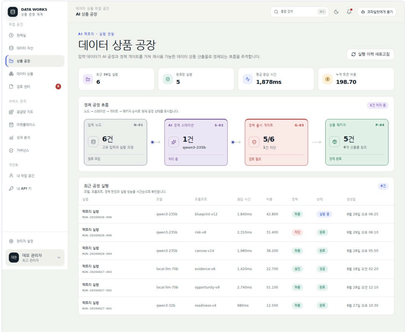
데이터 상품 공장 — AI 상품화 실행의 모델·비용·정책 판정과 상태를 확인한다
