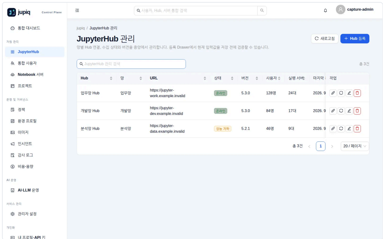
JupyterHub 관리 — 등록된 Hub의 상태·버전·사용자·실행 서버와 행별 작업 버튼
