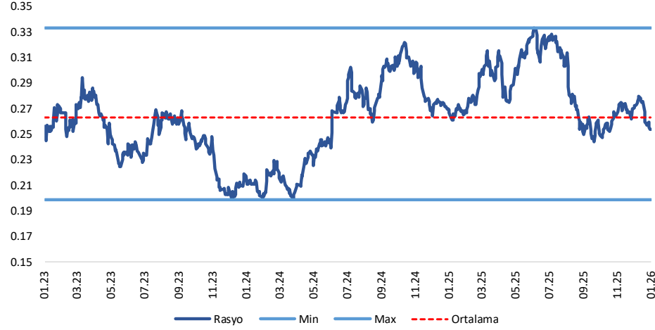
THYAO/PGSUS
