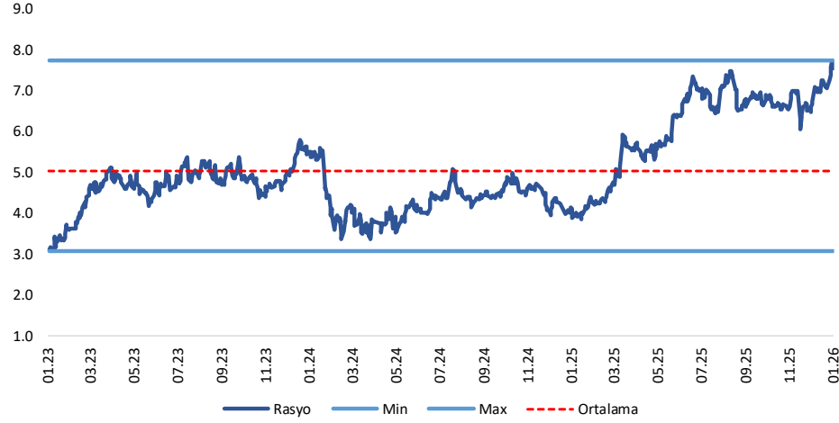
VESTL/ARCLK
