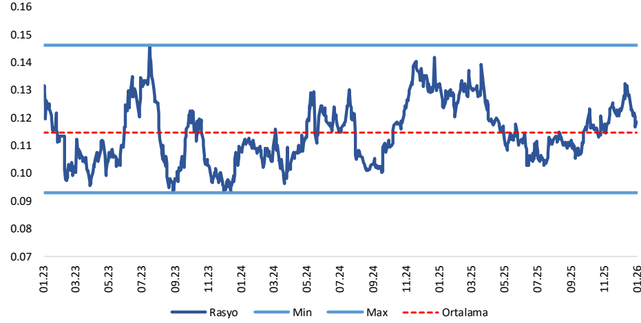
TUPRS/AYGAZ
