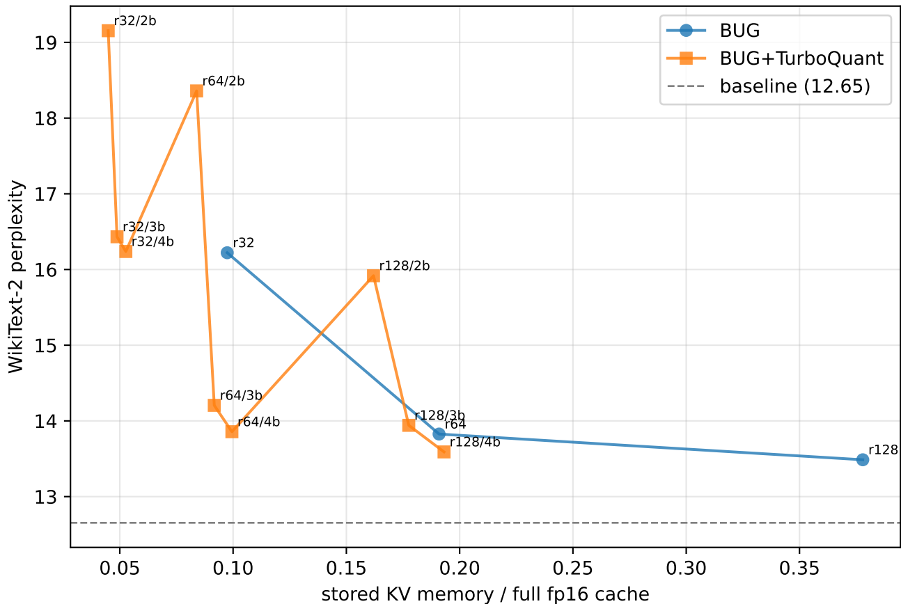
BUG vs BUG+TurboQuant — Llama-3.2-1B-Instruct, ctx 1024
