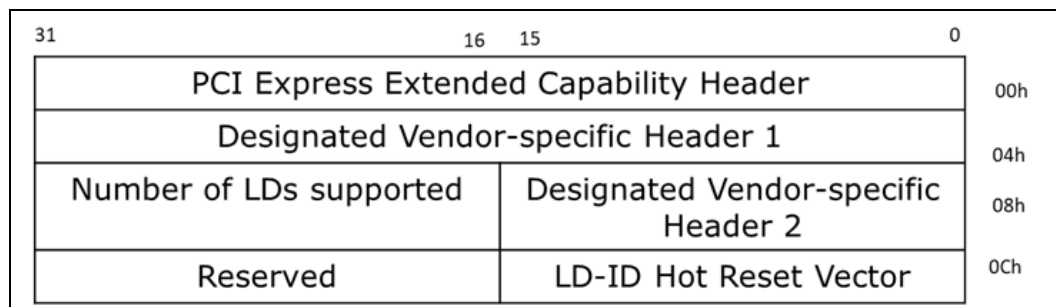
Figure 8-7. MLD DVSEC
