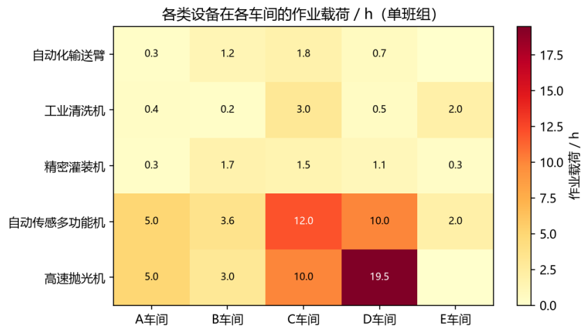
图 1 各类设备在各车间的作业载荷热力图（单班组，单位 h）
