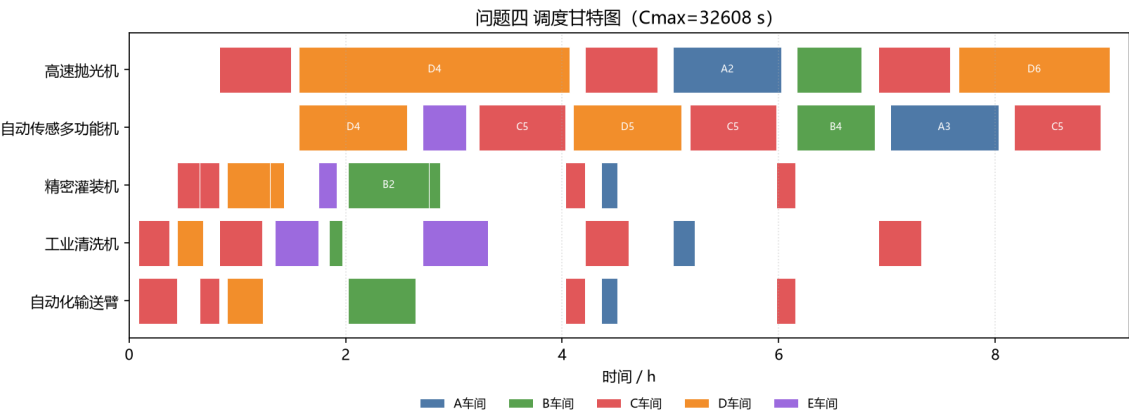
图 5 问题四调度甘特图 ( C_{\max} = 32608 s)
