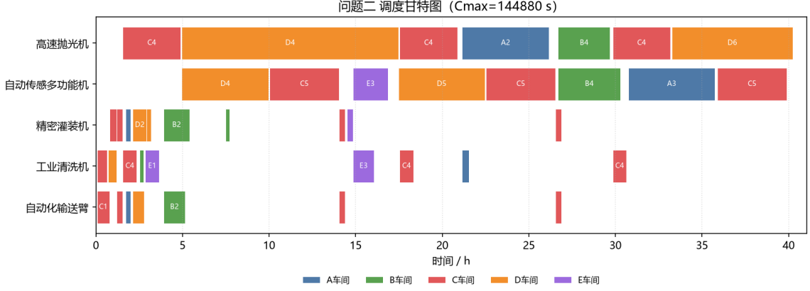
图 2 问题二调度甘特图 ( C_{\max} = 144880 \text{ s} )
