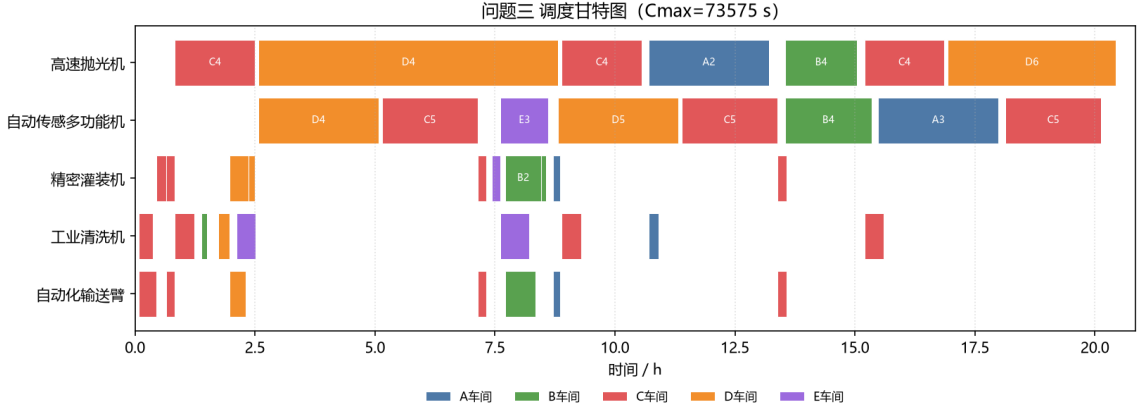
图 3 问题三调度甘特图 ( C_{\max} = 73575 s)
