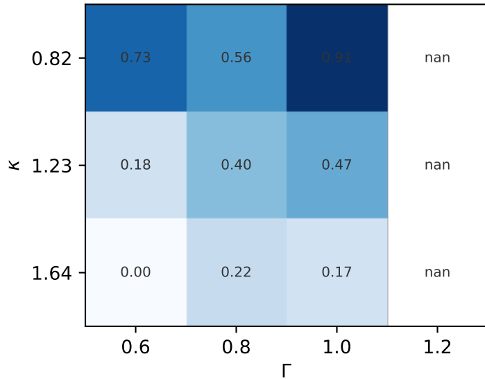
(b) tetraquark/meson [%]
