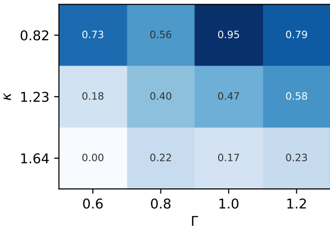
(b) tetraquark/meson [%]
