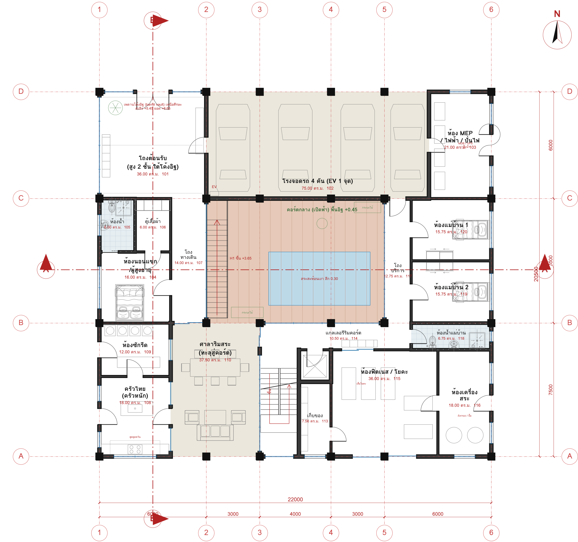
ผังพื้นชั้น 1 (FFL +0.45) 1:100
