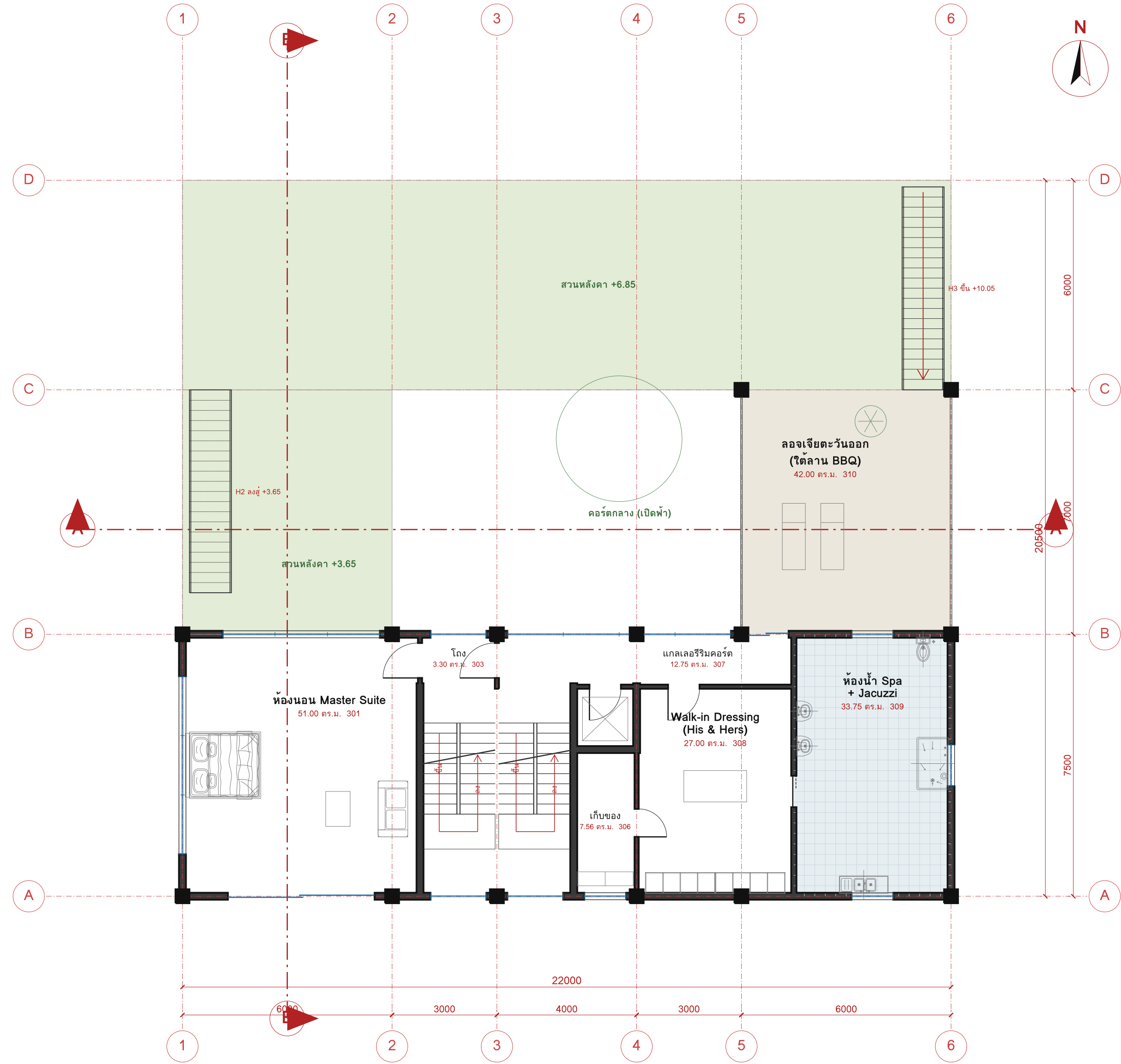
ผังพื้นชั้น 3 (FFL +6.85) 1:100
