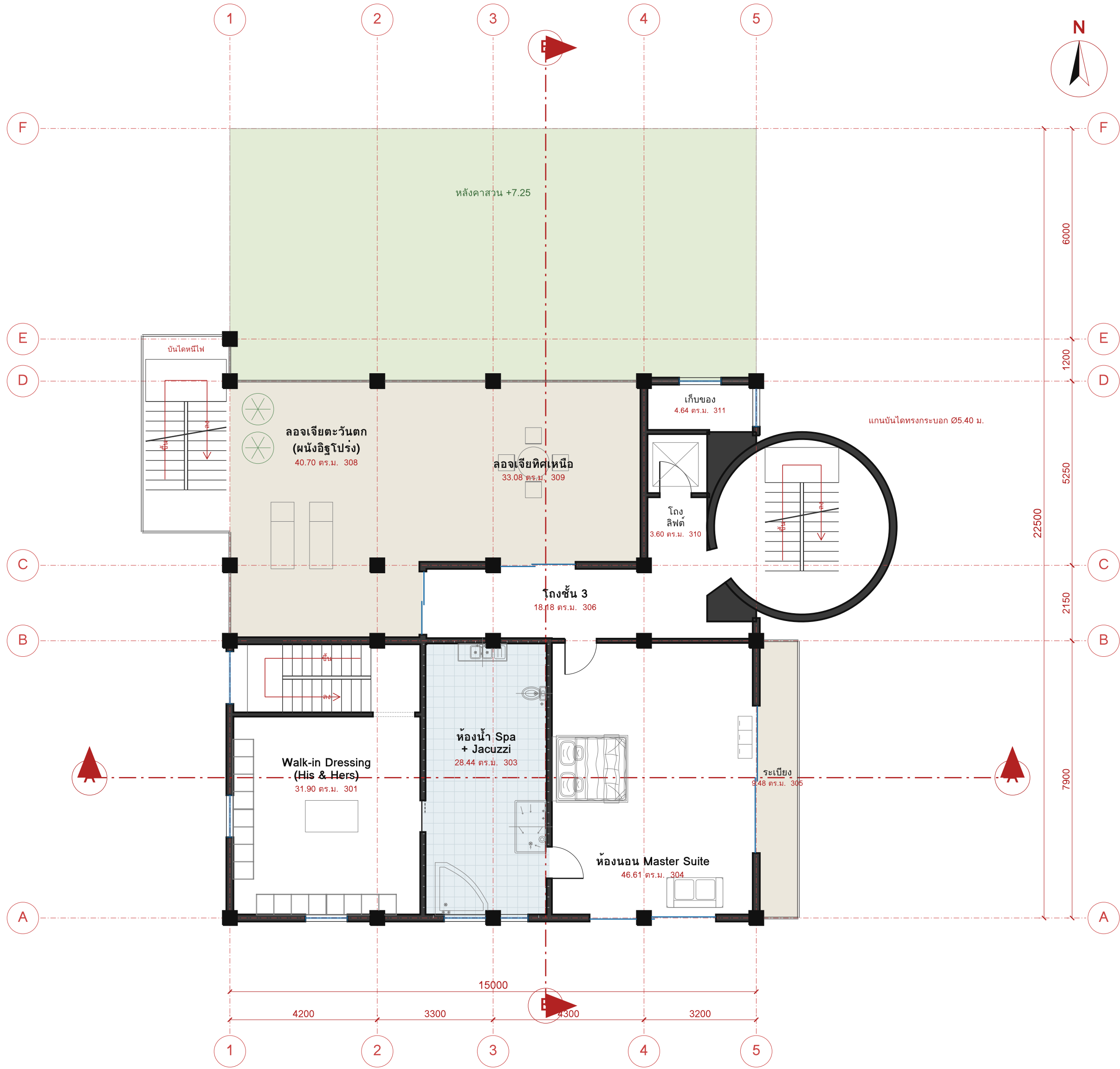
ผังพื้นชั้น 3 (FFL +7.25) 1:100
