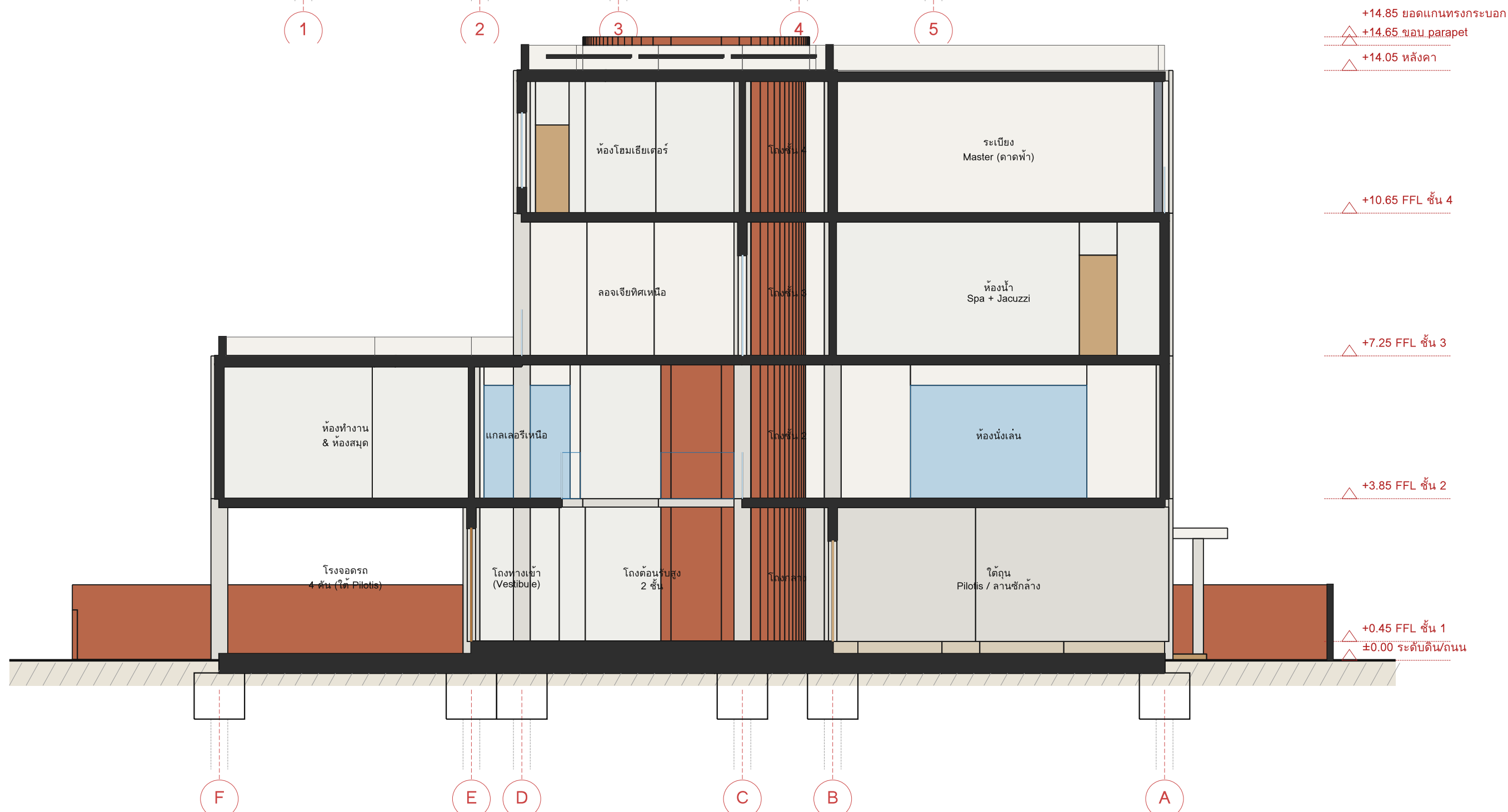
รูปตัด B-B (ตัดแนวเหนือ-ใต้ ผ่านใต้ถุน Pilotis-โถงต้อนรับสูง 2 ชั้น-โรงรถ / ห้องนั่งเล่น-ห้องทำงาน มองไปทิศตะวันออก เห็นแกนทรงกระบอก) 1:100
