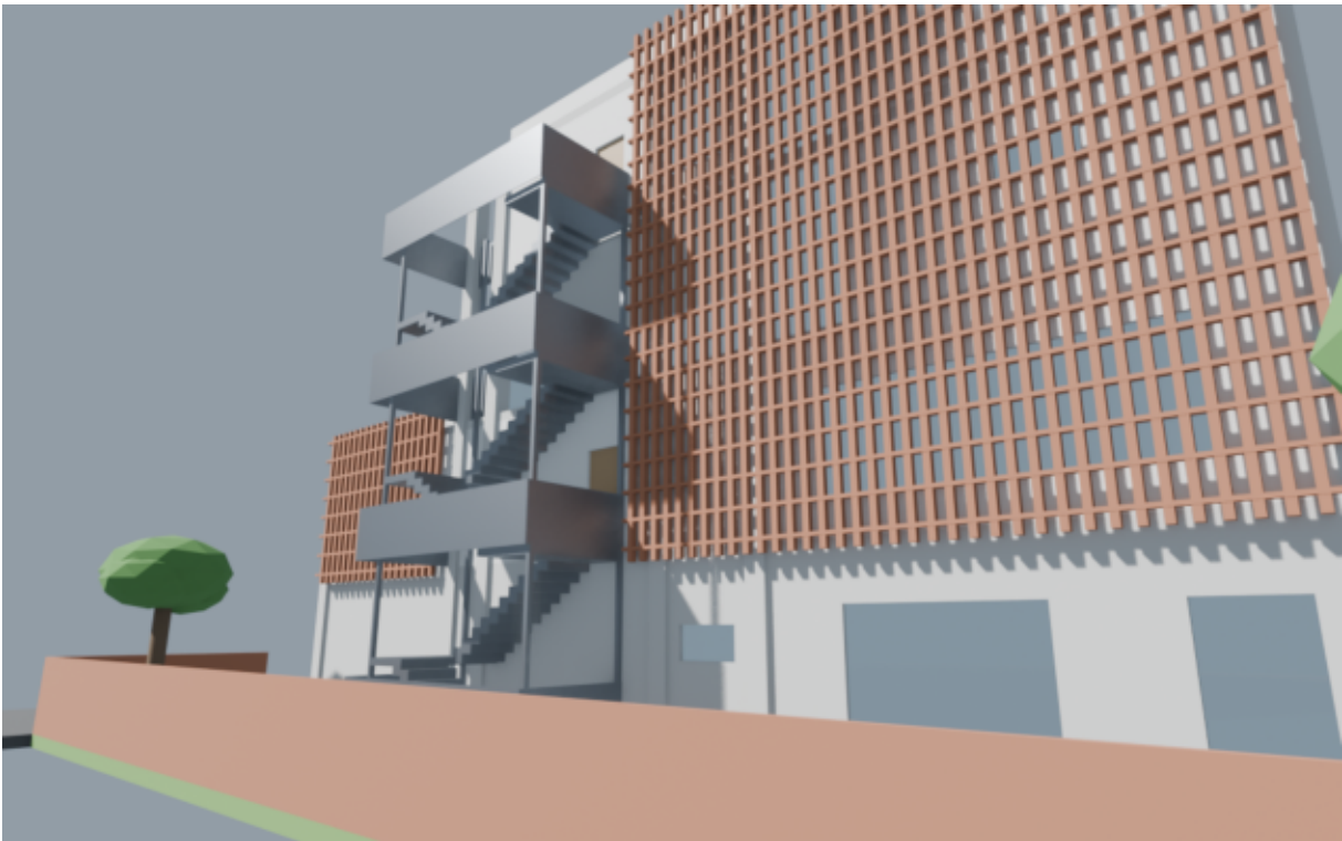
ผนังอิฐโปร่ง (ครึ่งอิฐ 115 มม. @290 + แบนบน @520) ทำหน้าอาคาร 0.34-0.45 ม.
