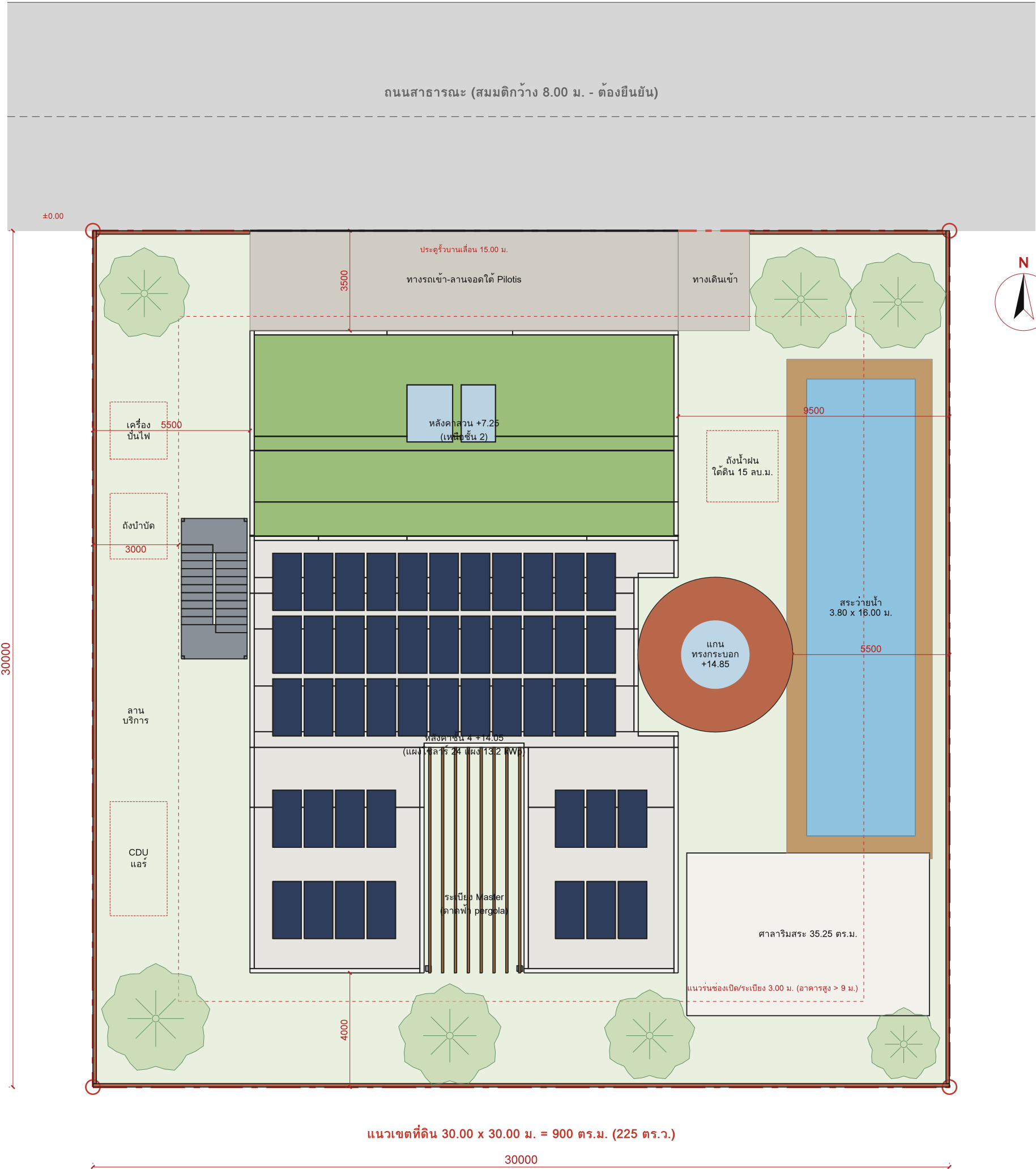
ผังบริเวณ SITE PLAN 1:150
