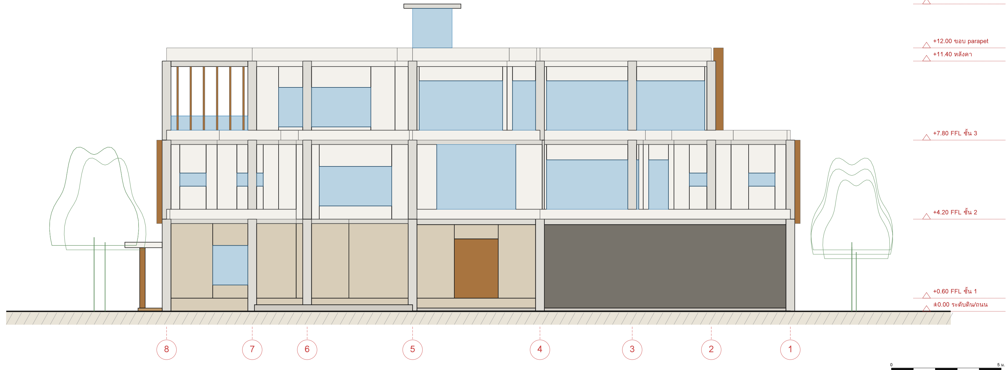
รูปด้านทิศเหนือ (ด้านถนน) 1:100
