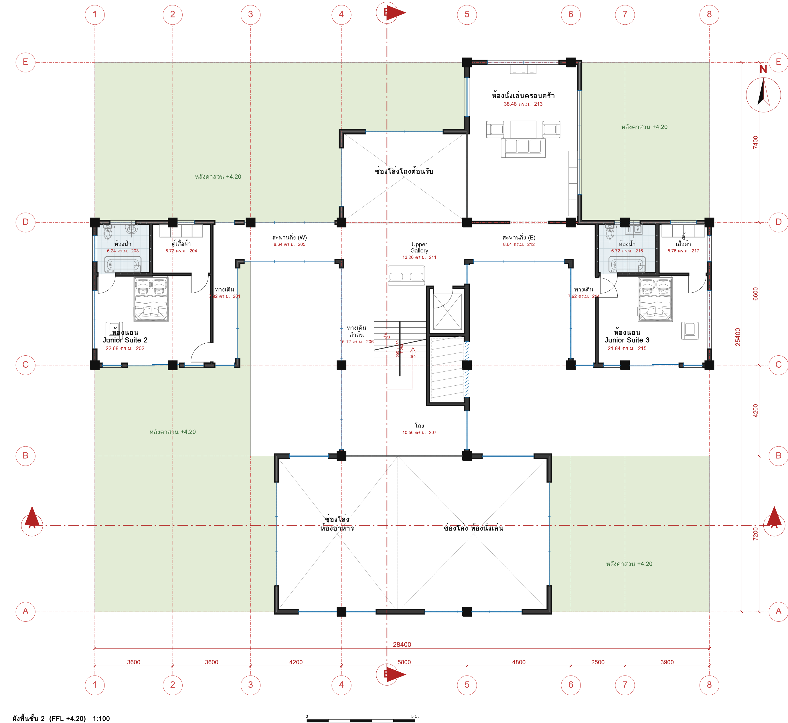
ผังพื้นชั้น 2 (FFL +4.20) 1:100
