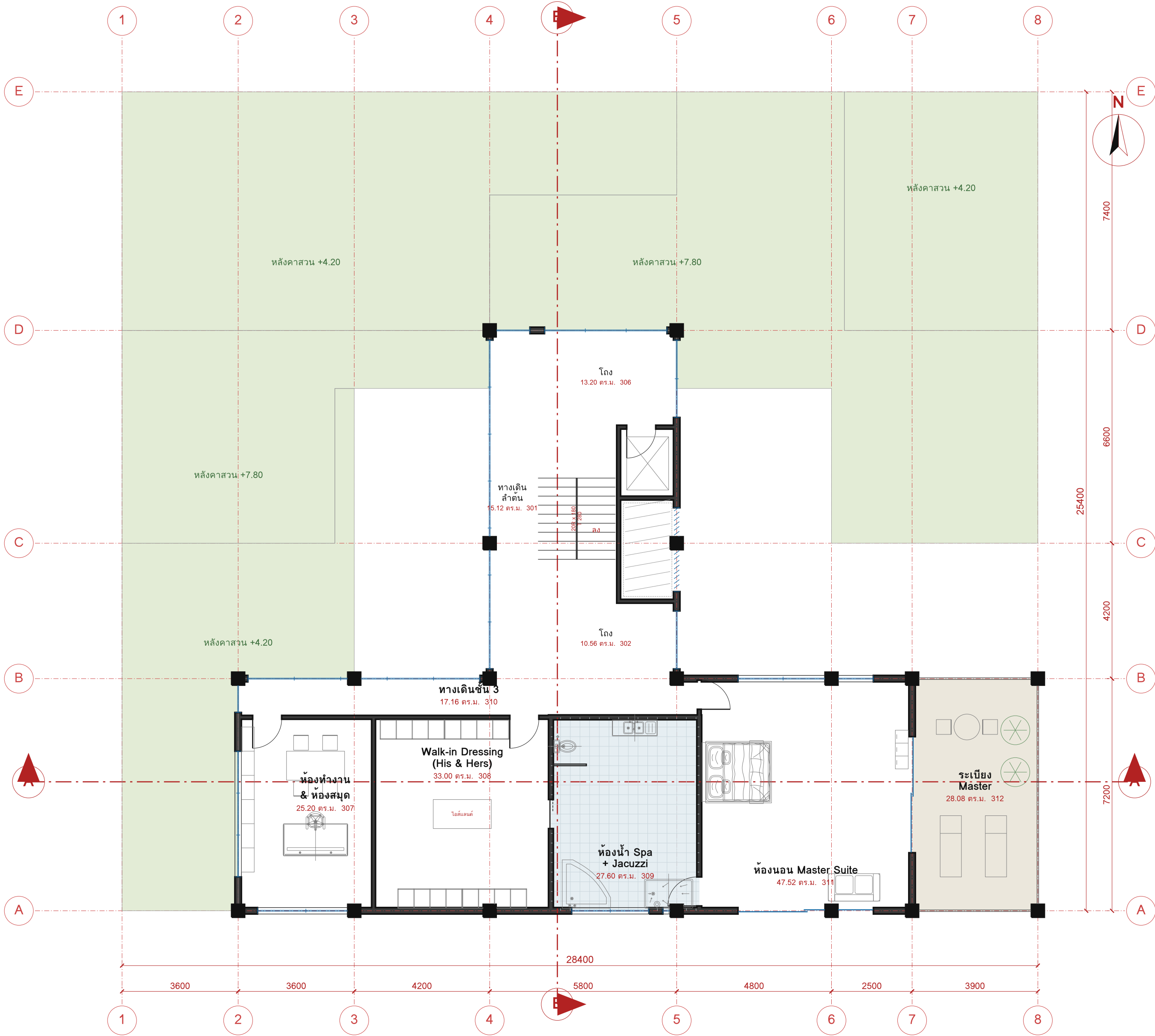
ผังพื้นชั้น 3 (FFL +7.80) 1:100
