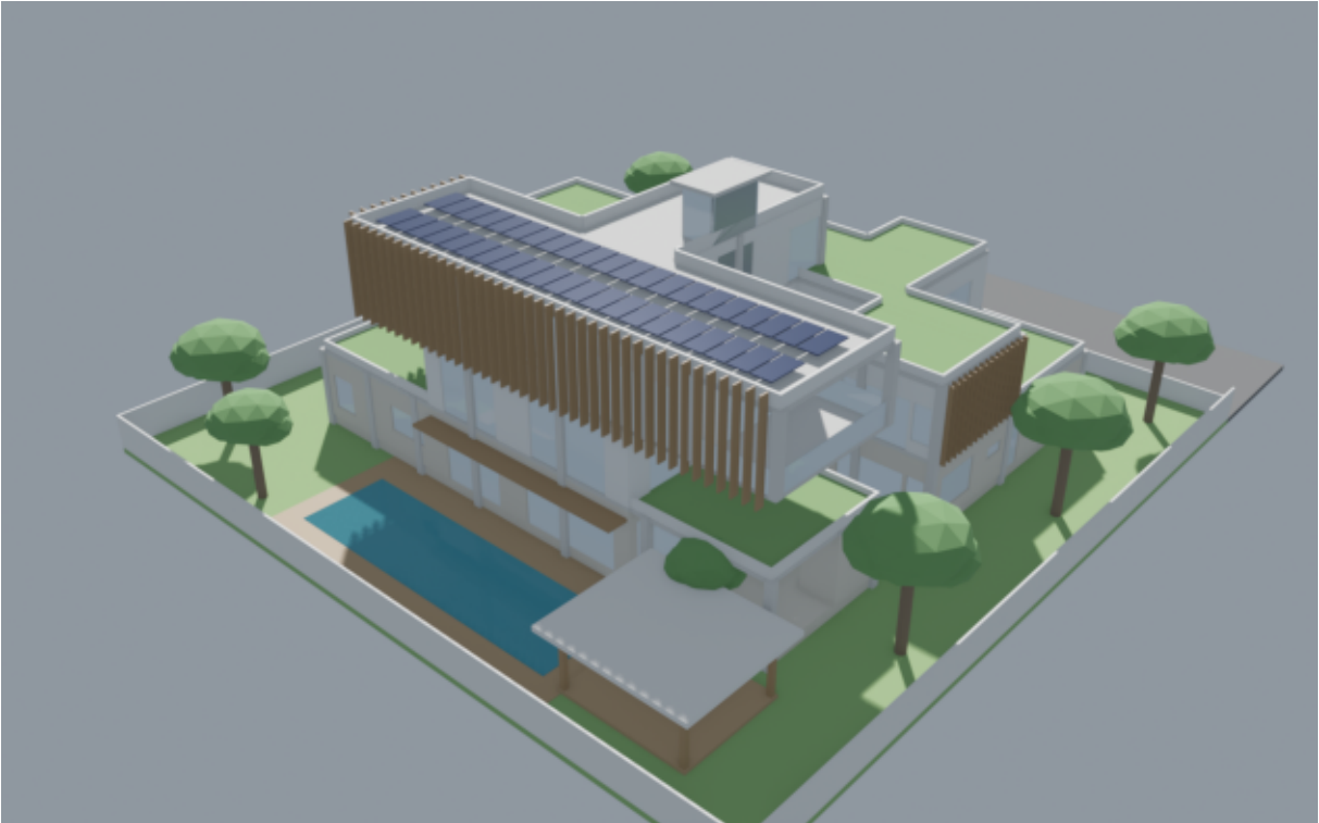
มุมมองทางอากาศ ทิศตะวันออกเฉียงใต้ — Crown bar ชั้น 3 ห่อด้วยครีปไม้ (CACTUS skin) + แผงโซลาร์ 23.1 kWp
