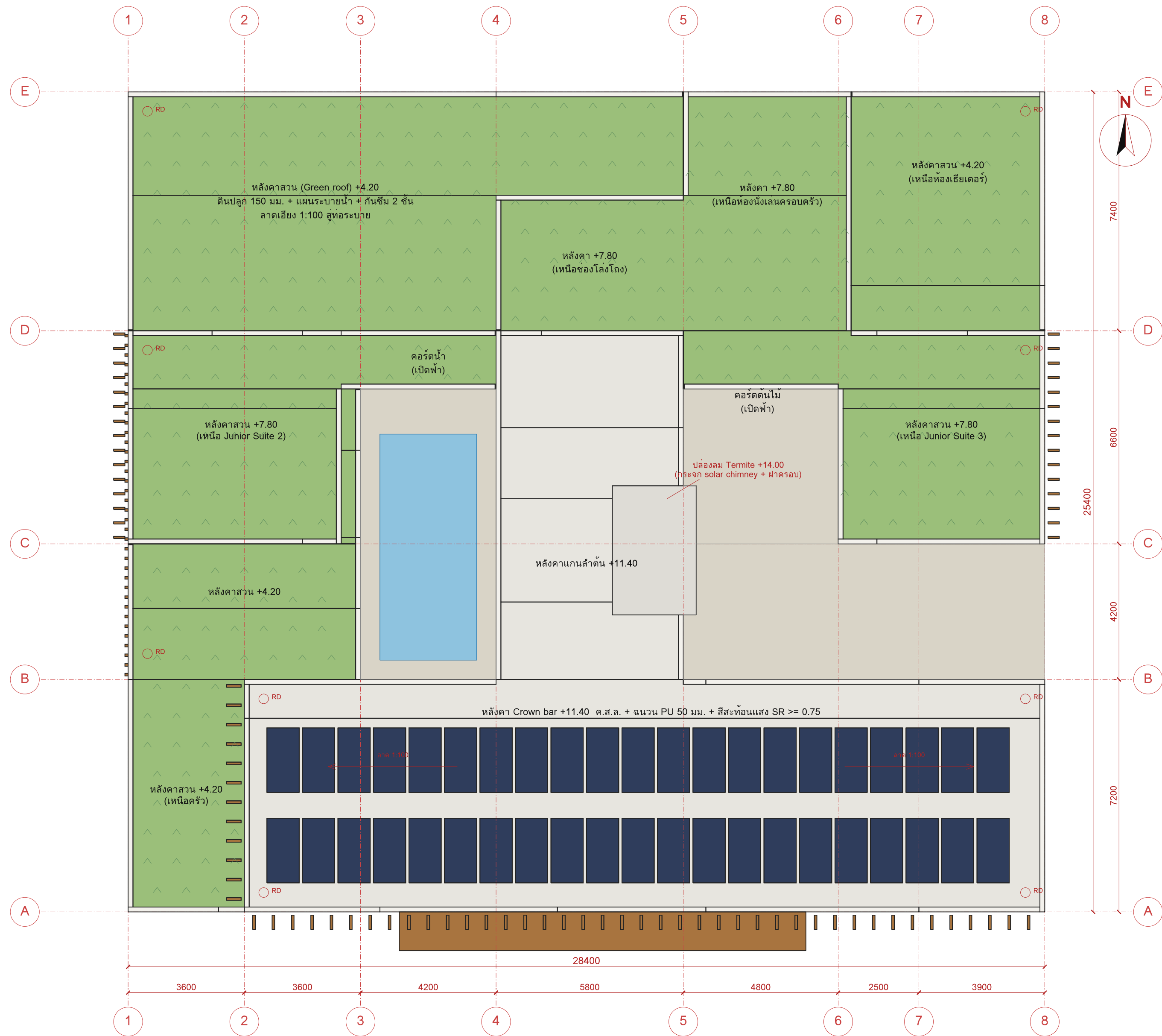
แปลนหลังคา ROOF PLAN 1:100
