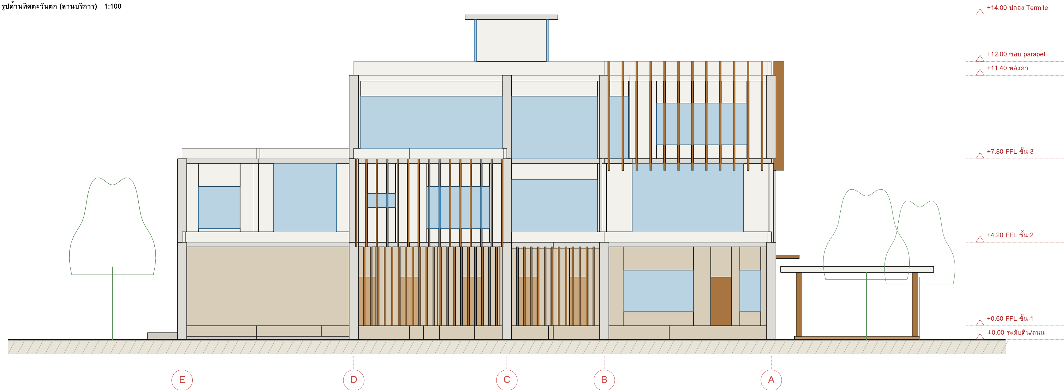
รูปด้านทิศตะวันตก (ลานบริการ) 1:100
