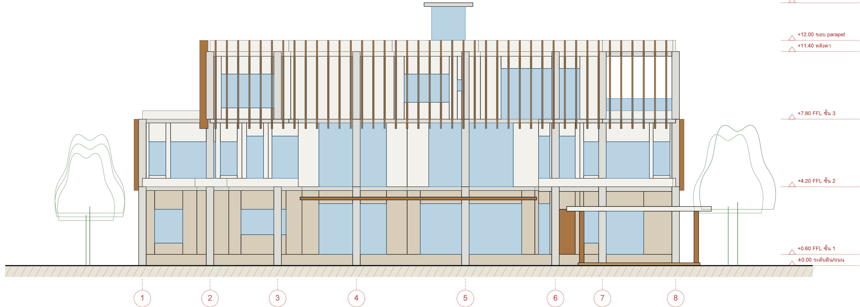
รูปด้านทิศใต้ (มองจากสวน/สระ) 1:100
