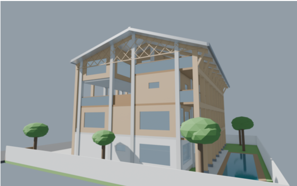
หน้าจั่วทิศตะวันตก — ระแนงไม้ทแยง คอร์ตแสงหัวท้าย และเพรชไม้ glulam ด้านใต้
