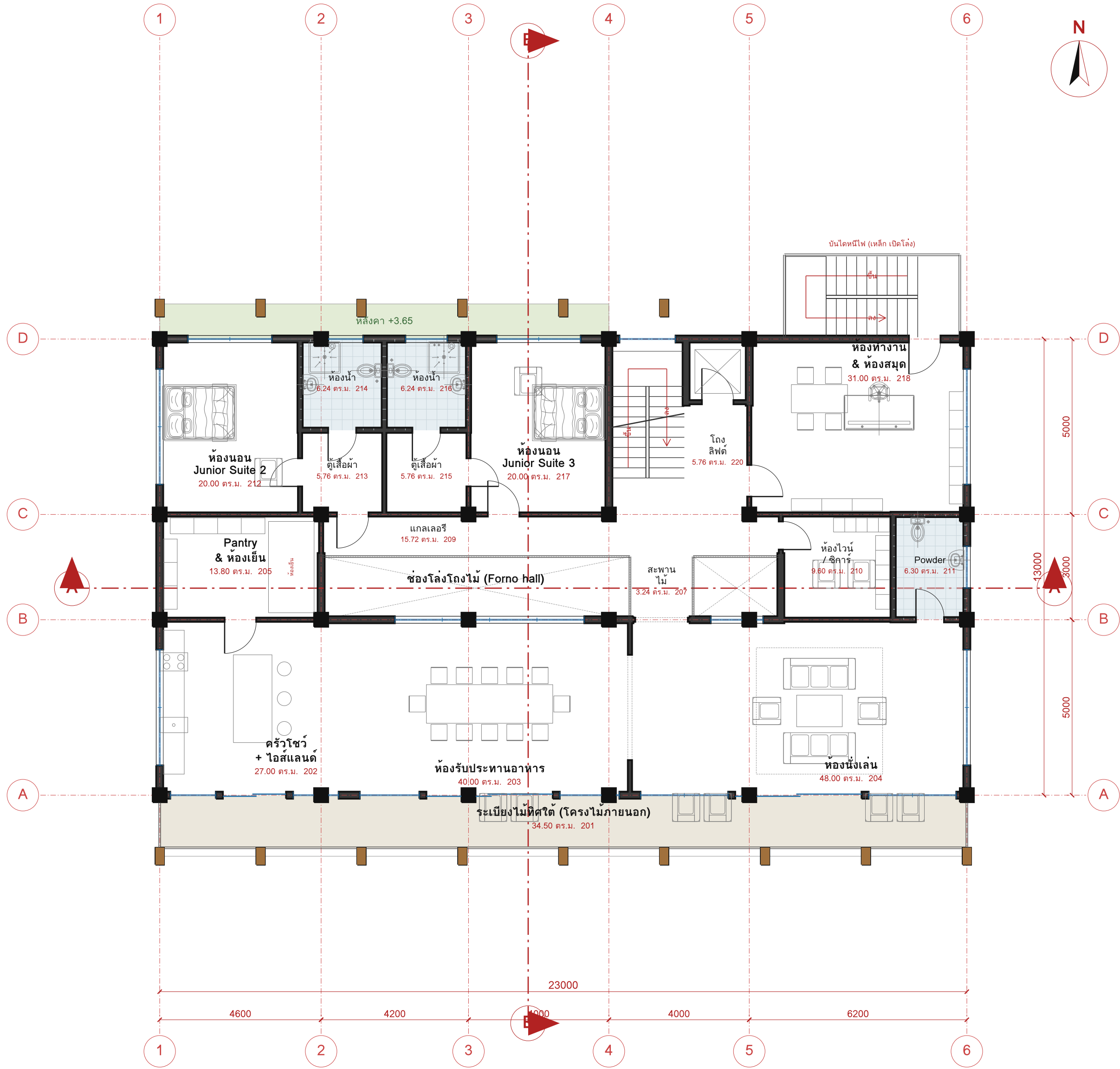
ผังพื้นชั้น 2 (FFL +3.65) 1:100
