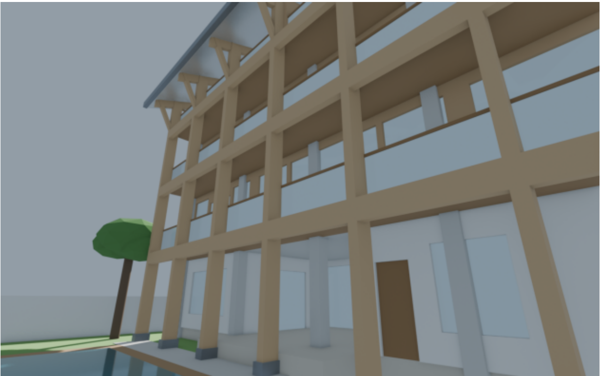
จากสวนสระทิศใต้ — เสาโครงไม้ภายนอก + ค้ำเชิงรับชายคา 3.00 ม. ระเบียงไม้ทุกชั้น ผนังกระจกเต็มบาน
