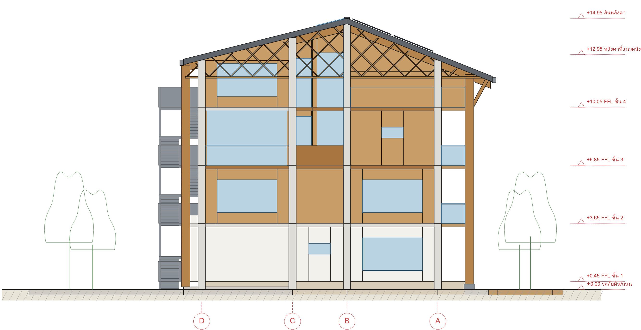
รูปด้านทิศตะวันตก (หน้าจั่ว + ระแนงไม้ทแยง) 1:100
