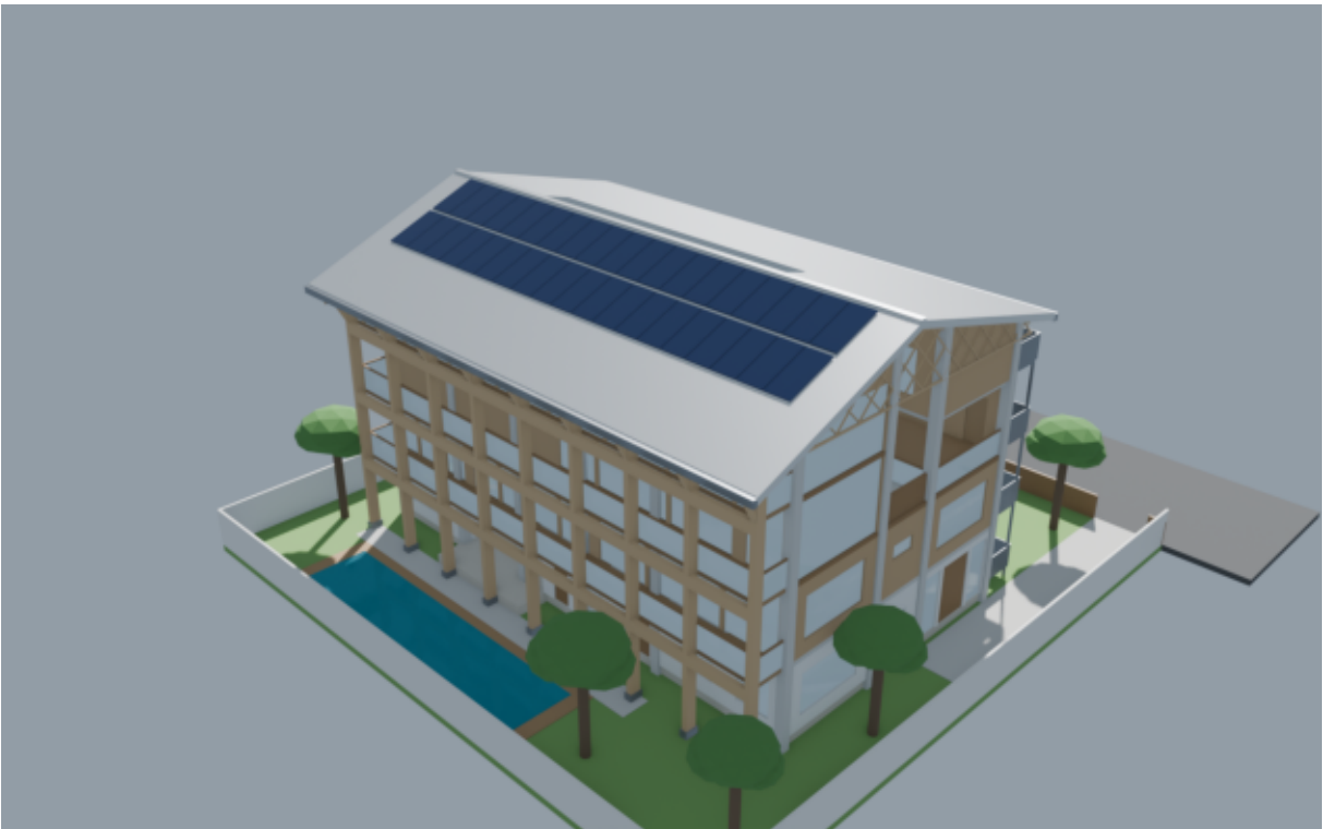
มุมมองทางอากาศ ทิศตะวันออกเฉียงใต้ — หลังคาจั่วไม้สมมาตรคลุมทั้ง 23.00 x 13.00 ม. แผงโซลาร์ลาดใต้ ช่องแสงชั้นหลังคา
