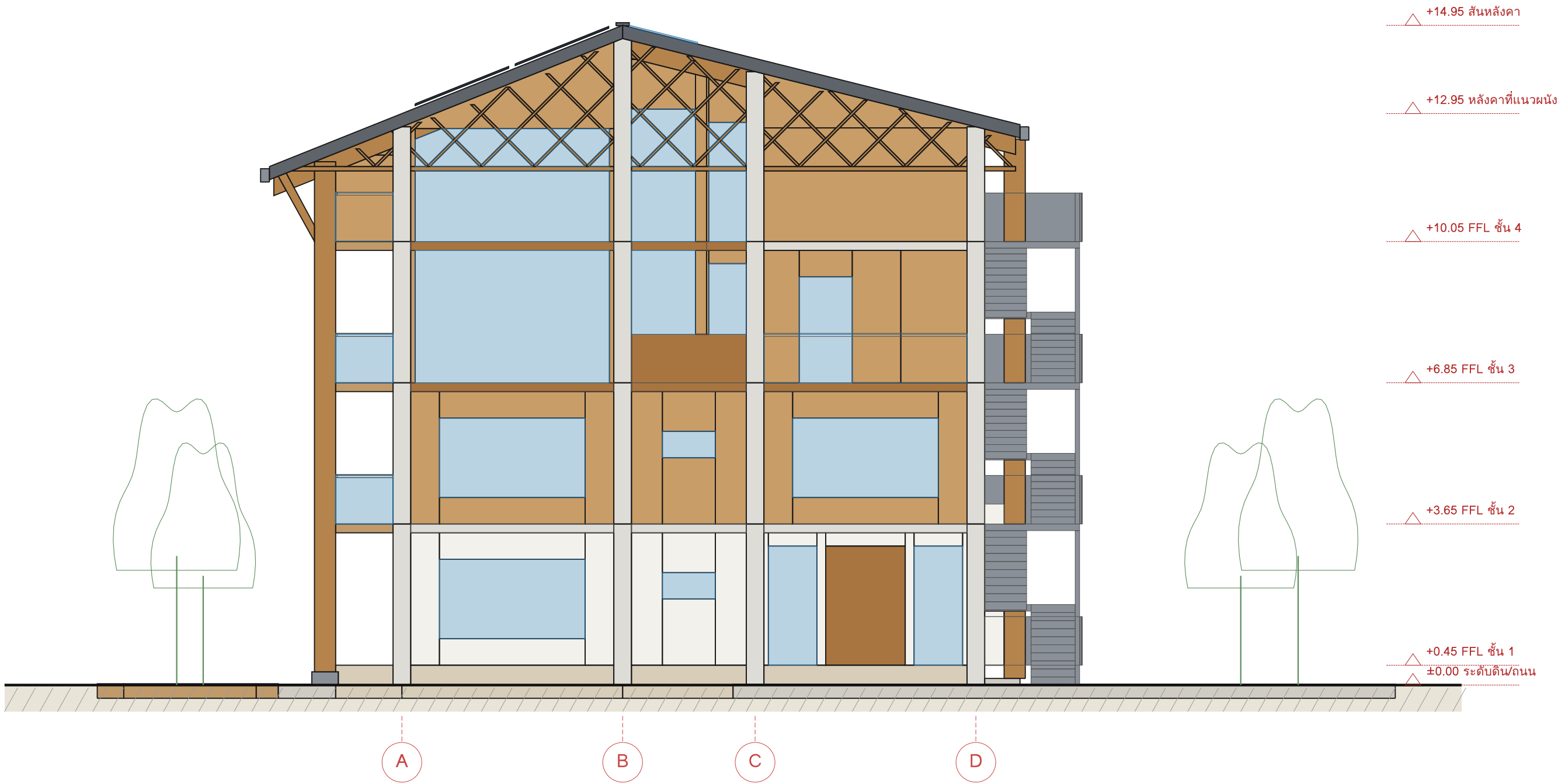
รูปด้านทิศตะวันตก (หน้าจั่ว + ระแนงไม้ทแยง) 1:100
