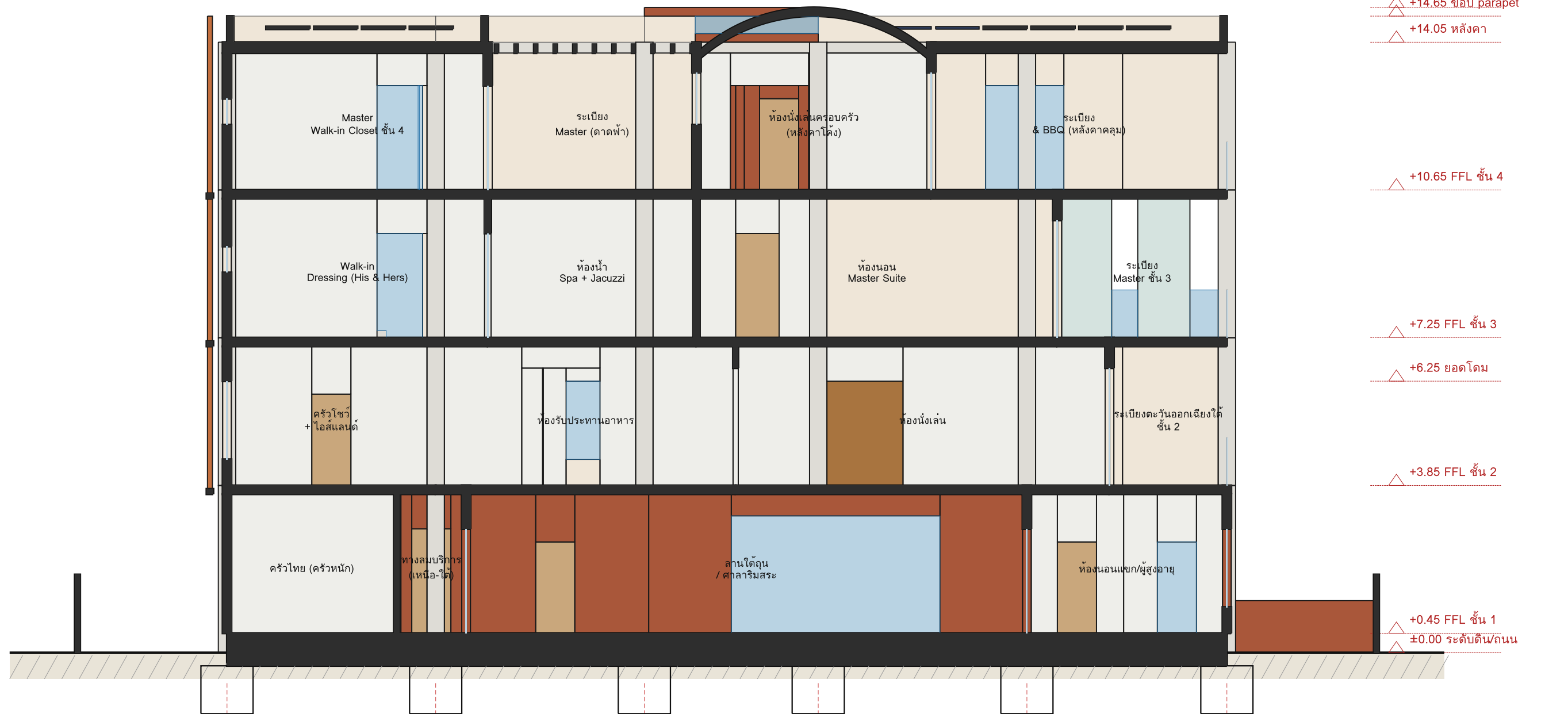
รูปตัด B-B (ตัดแนวเหนือ-ใต้ ผ่านโดมอิฐ-โก่งทางเข้า-โก่งกลาง-ลานใต้ถุน / ห้องนั่งเล่น-ทางเดิน-ห้องไวน์ / ห้องนอน Master-ลงเจีย / BBQ-ห้องเสิร์ฟเตอร์ มองไปทิศตะวันออก) 1:100
