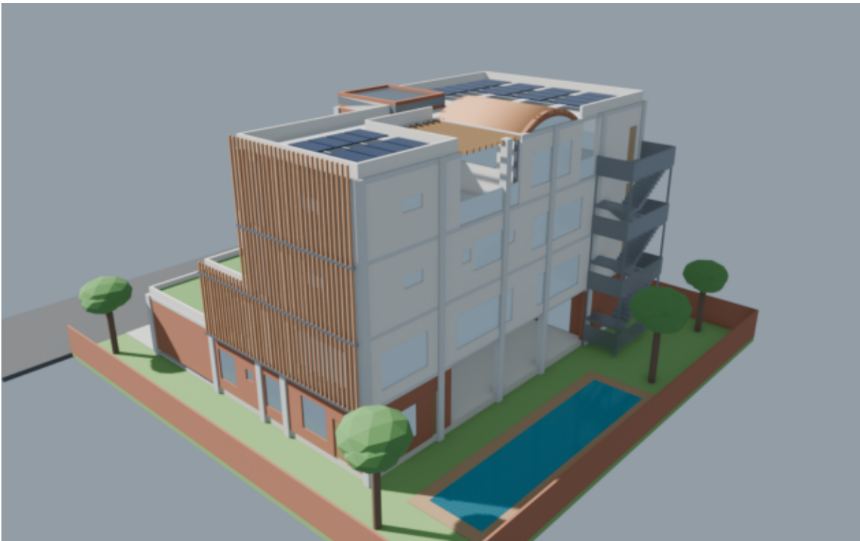
มุมมองทิศตะวันตกเฉียงใต้ — คริบดินเผาทิศตะวันตก (ปีงแดดบ่าง) ฐานอิฐชั้น 1 สระ 14.00 x 3.00 ม.
