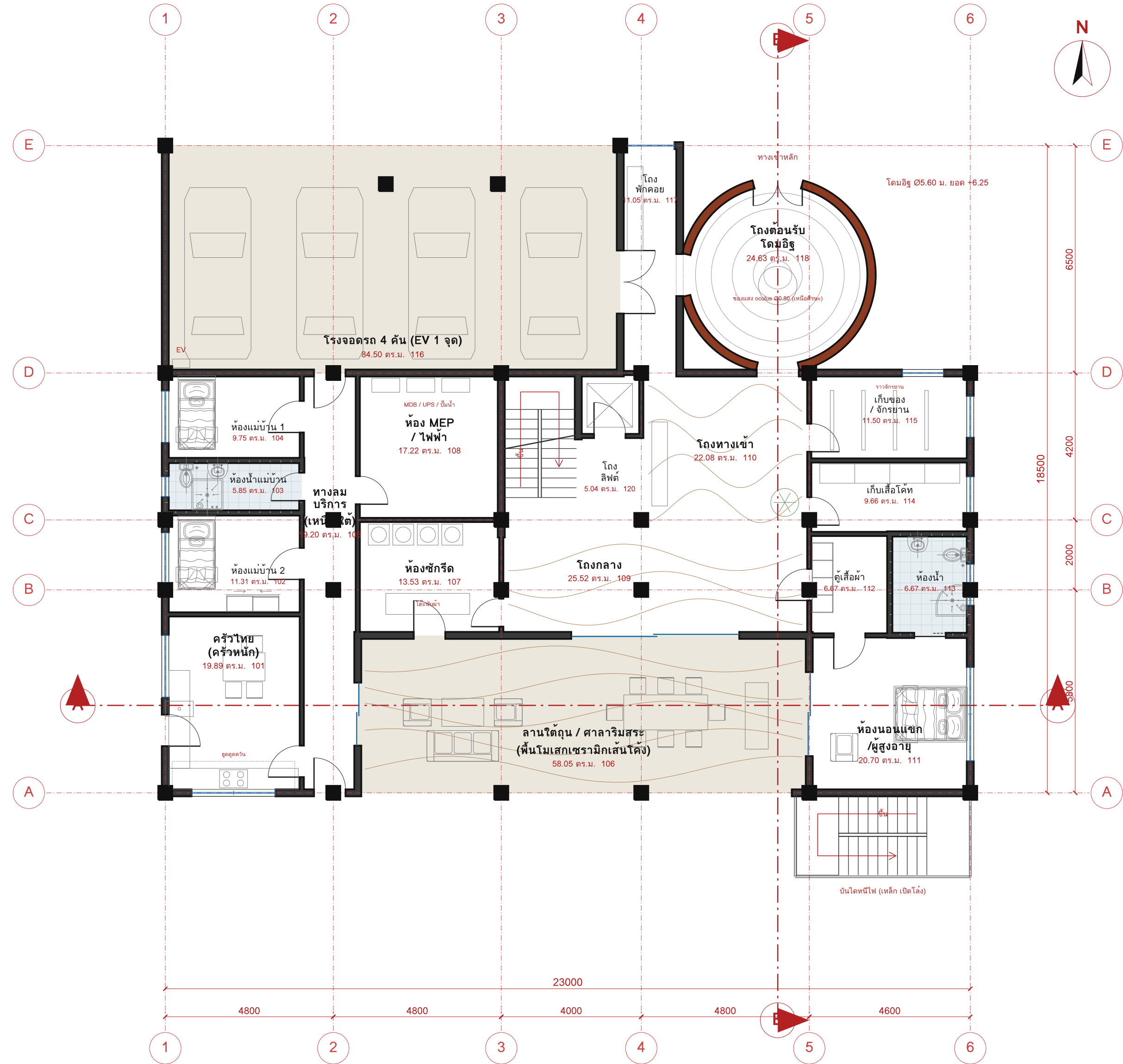
ผังพื้นชั้น 1 (FFL +0.45) 1:100
