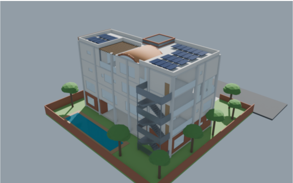
มุมมองทางอากาศ ทิศตะวันออกเฉียงใต้ — แท่งอาคาร 23.00 x 12.00 ม. หลังคาโค้งดินเผา ปล่องอิฐ และบันไดหนีไฟเหล็ก
