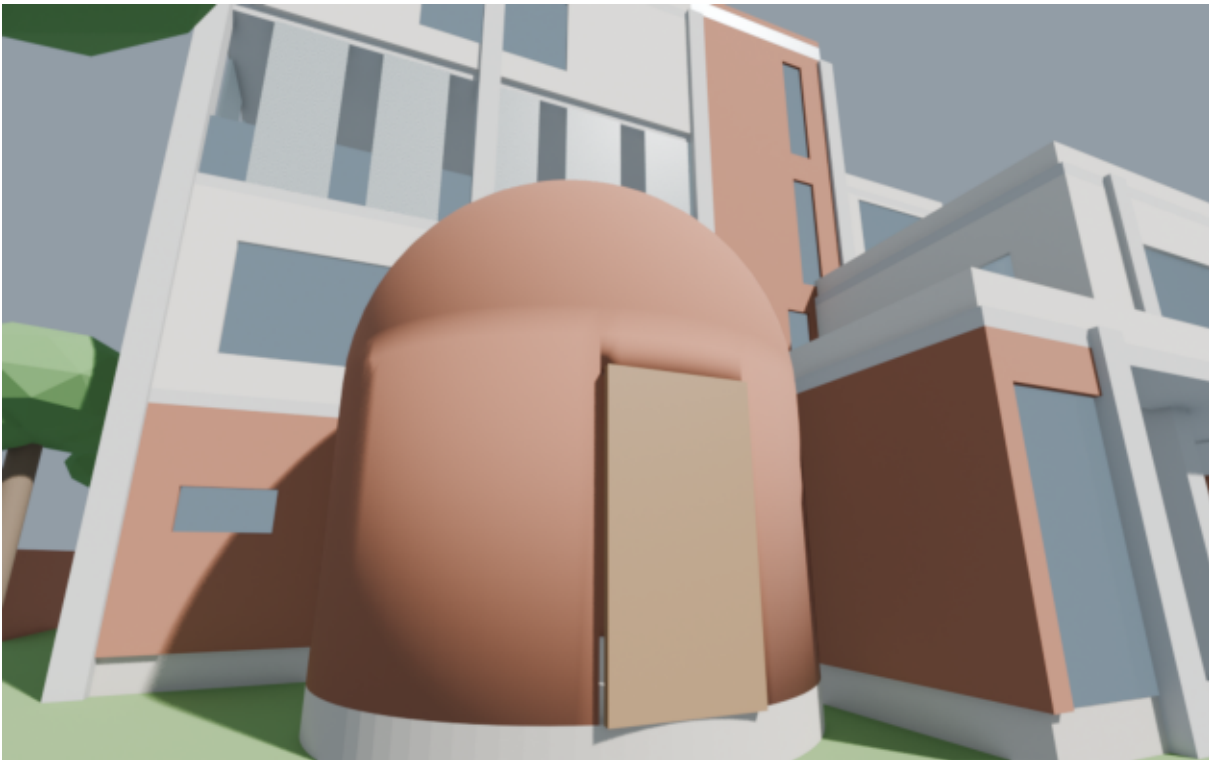
ทางเข้าโดมอิฐ Ø5.60 ม. ยอด +6.25 ช่องแสง oculus ด้านบน ปล่องอิฐด้านหลัง
