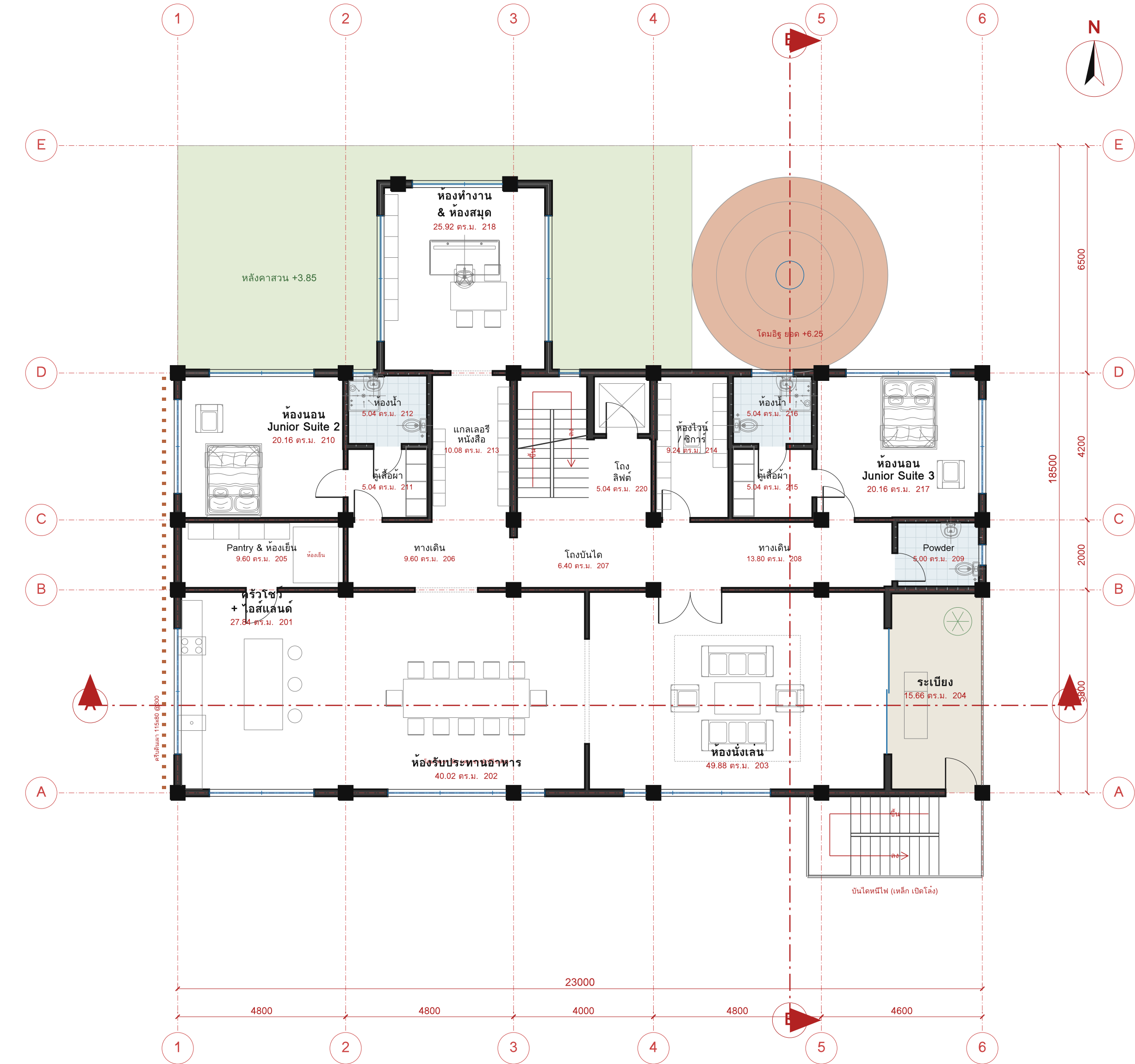
ผังพื้นชั้น 2 (FFL +3.85) 1:100
