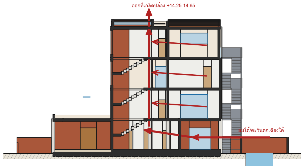
ลูกศร = เจตนารการออกแบบ (ลมปะจำกรุงเพทฯ ฤดูร้อน S/SW, ทวนำ NE) — ยังไม่ได้พิสูจน์ด้วย CFD/การจำลองความร้อน
