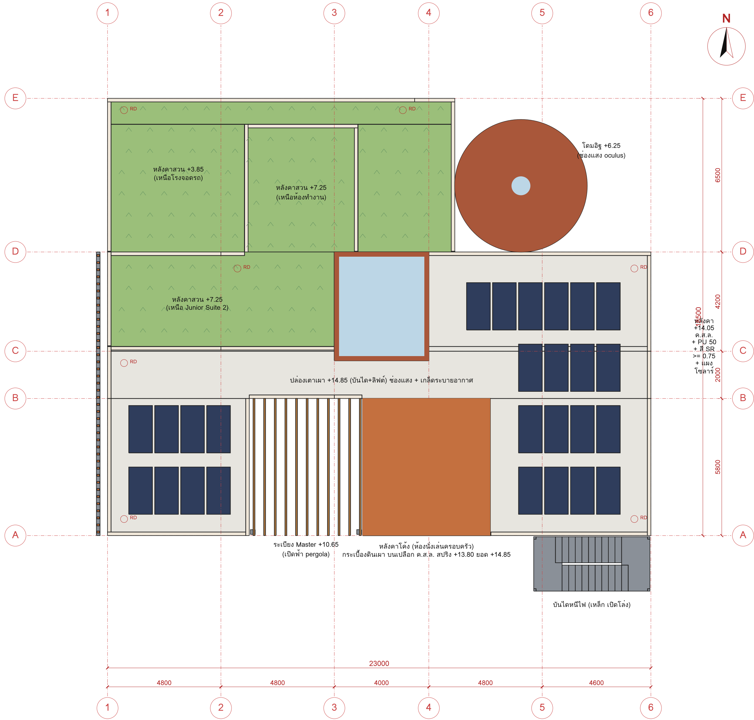
แปลนหลังคา ROOF PLAN 1:100
