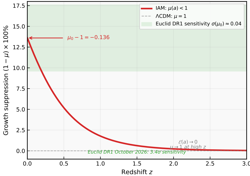
(d) Observational Consequence: Growth Suppression
