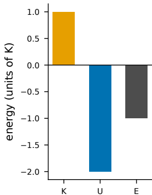
a Virial: U = -2K , E = -K
