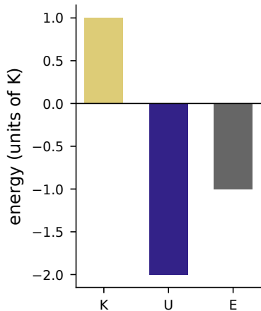
a Virial: U = -2K , E = -K
