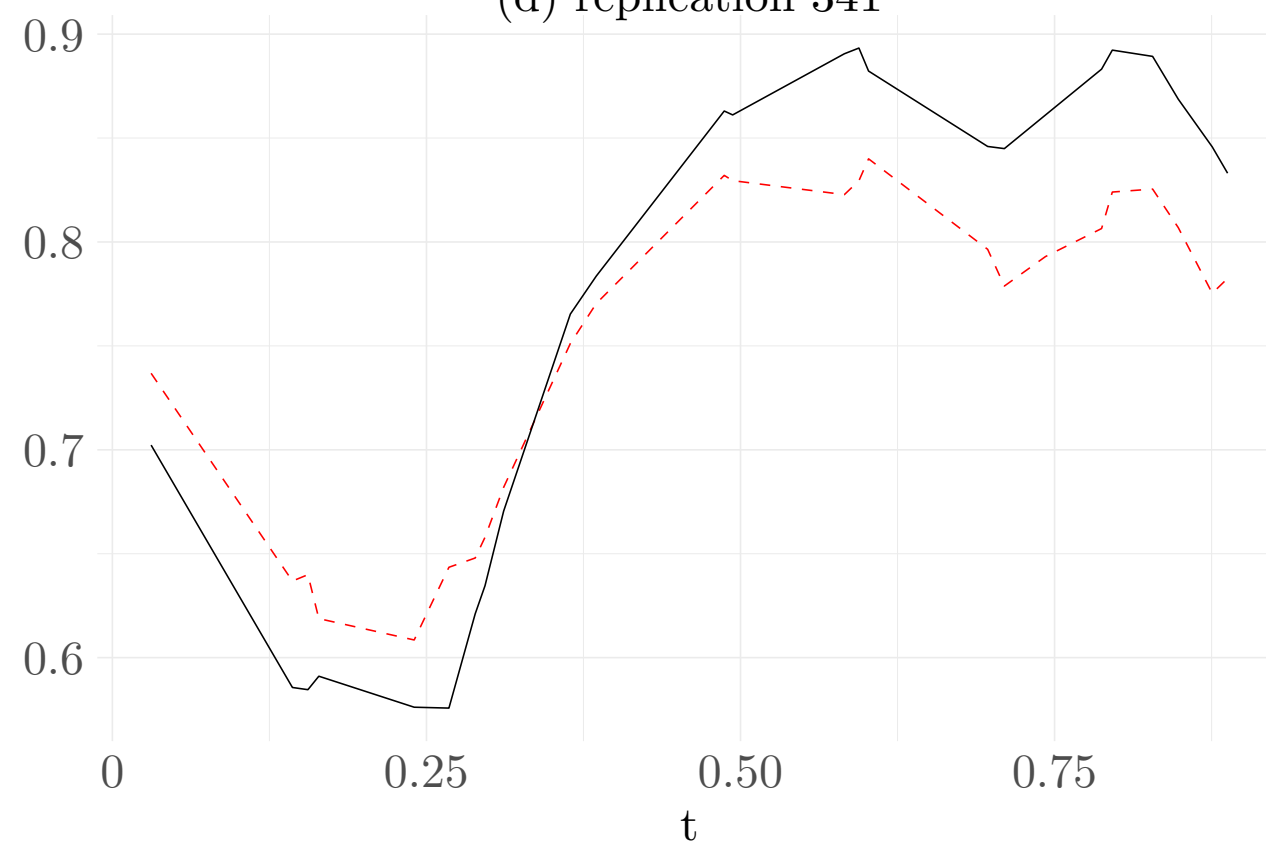
(d) replication 341
