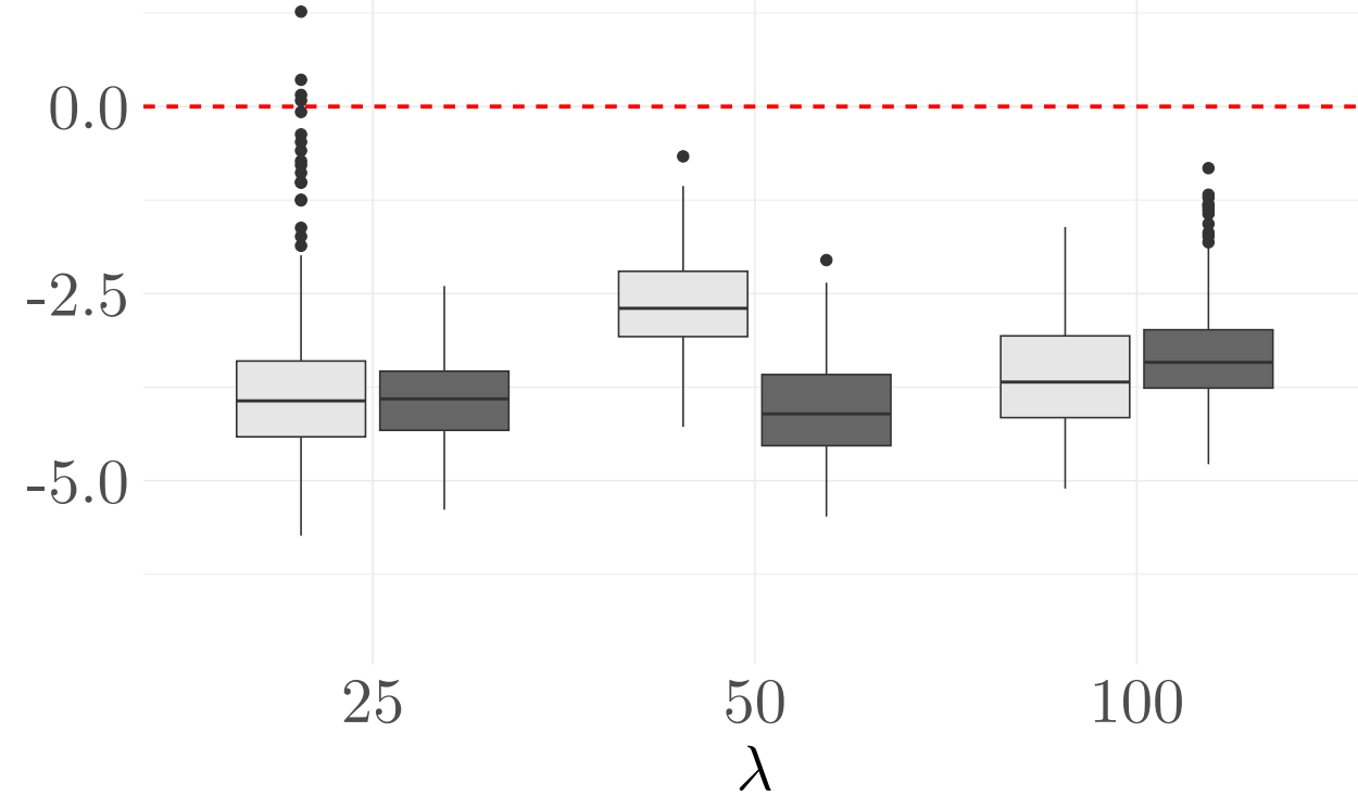
(d) ISE ratio w.r.t. RP20 under \mathcal{T}_{n_0}^{3/4}
