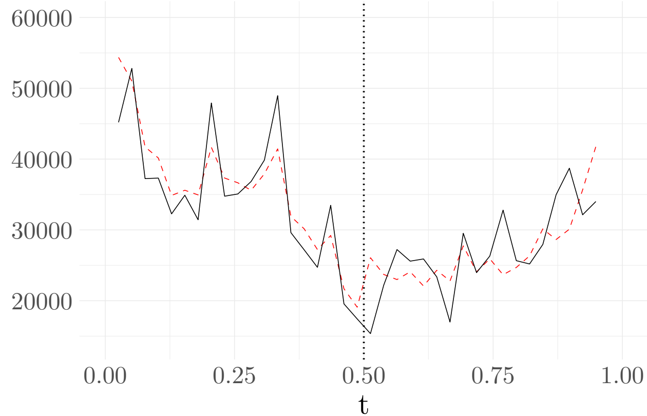
(d) Facebook stock volume \mathcal{T}_{n_0}^1
