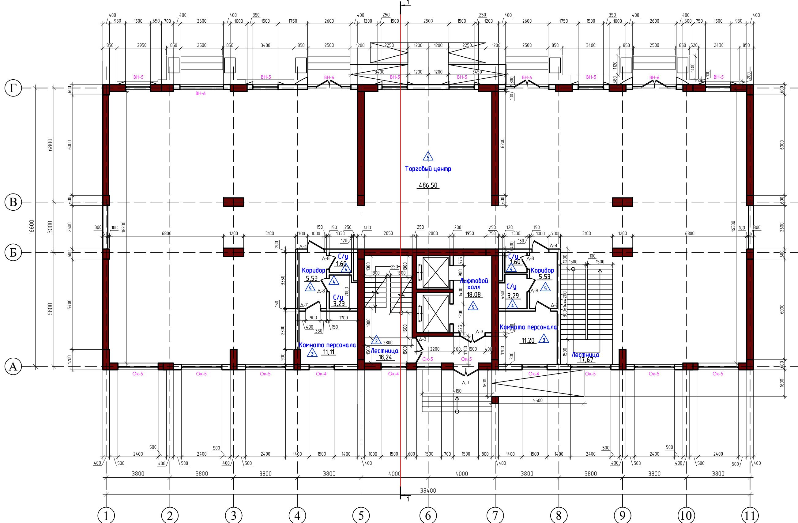
Экспликация помещений
