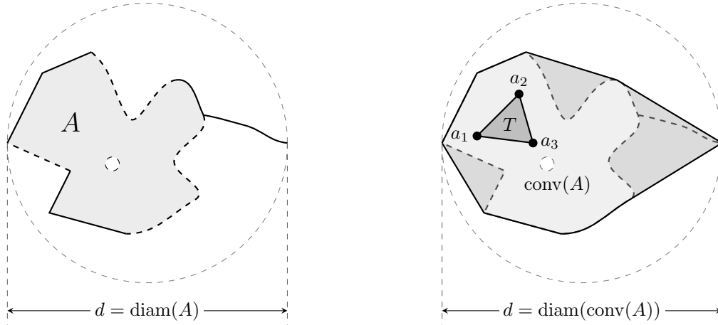
(a) Conjunto medible A \subset \mathbb{R}^2 con diámetro d = \text{diam}(A) marcado. (b) Envoltente convexa de A con el triángulo T = \text{conv}(\{a_i\}_{i=1}^3) \subset \text{conv}(A) .
